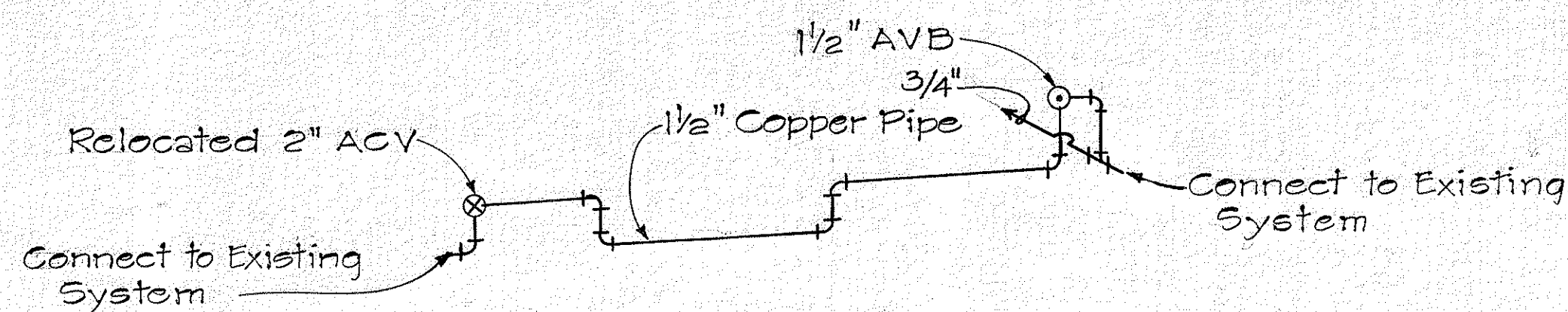
PIPE DIAGRAM STA. 0+58 TO STA. 2+00
