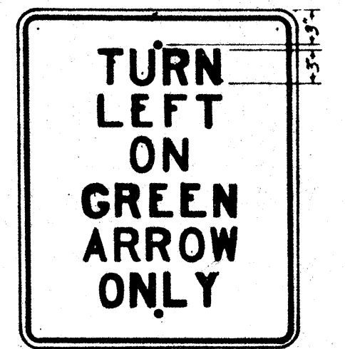
R-107-A 24" x 30"
