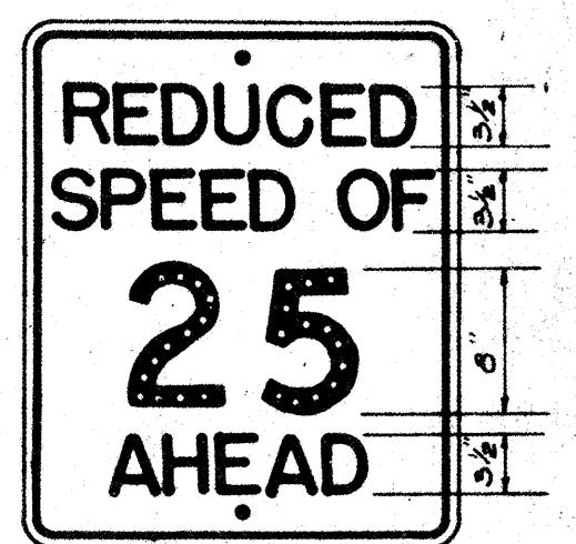
R-104-A 24" x 30"
