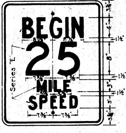
R-105-A 24" x 30"
