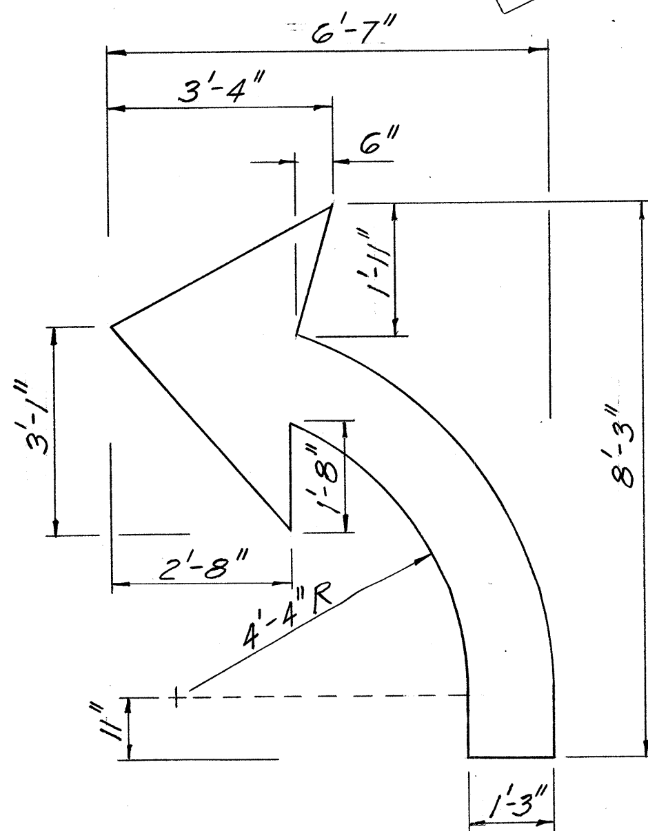
PAVEMENT ARROW Scale: 1/2" = 1'-0"
