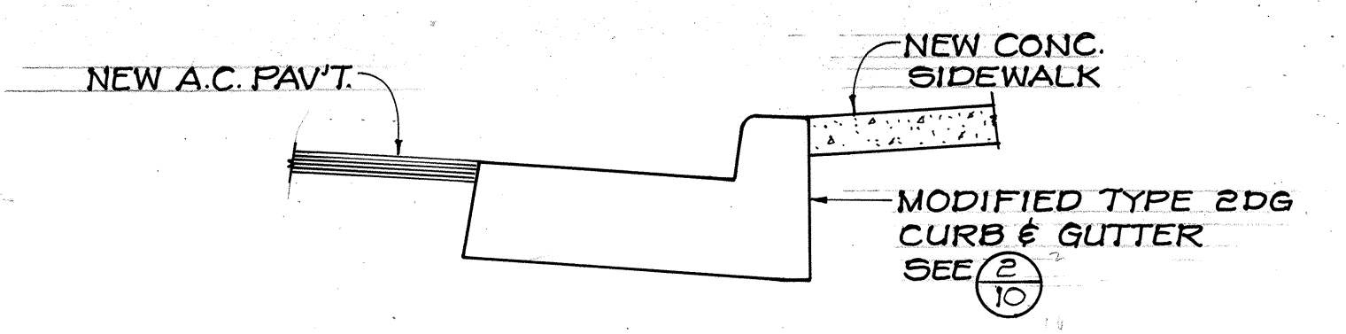
A SECTION SCALE: 3/4" = 1'-0"
