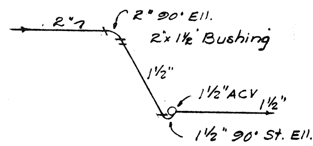
DETAIL 5-A
