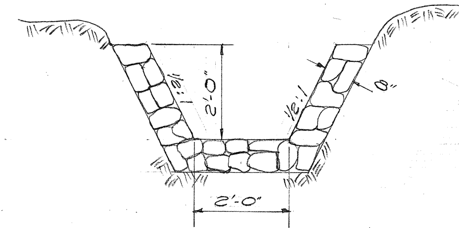
SECTION "C-C" SCALE: 1/2" = 1'-0"
