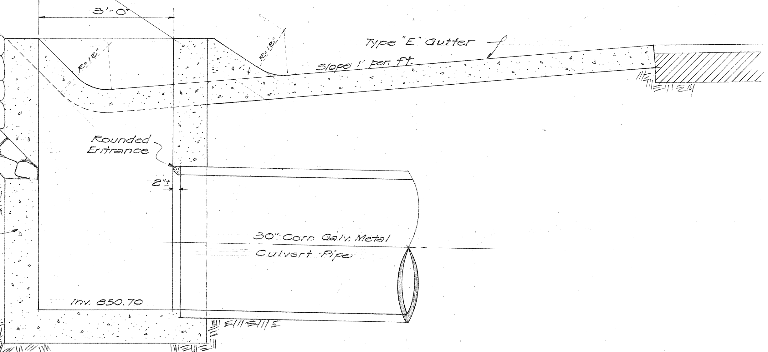
SECTION "C-C" SCALE: 1/2" = 1'-0"
