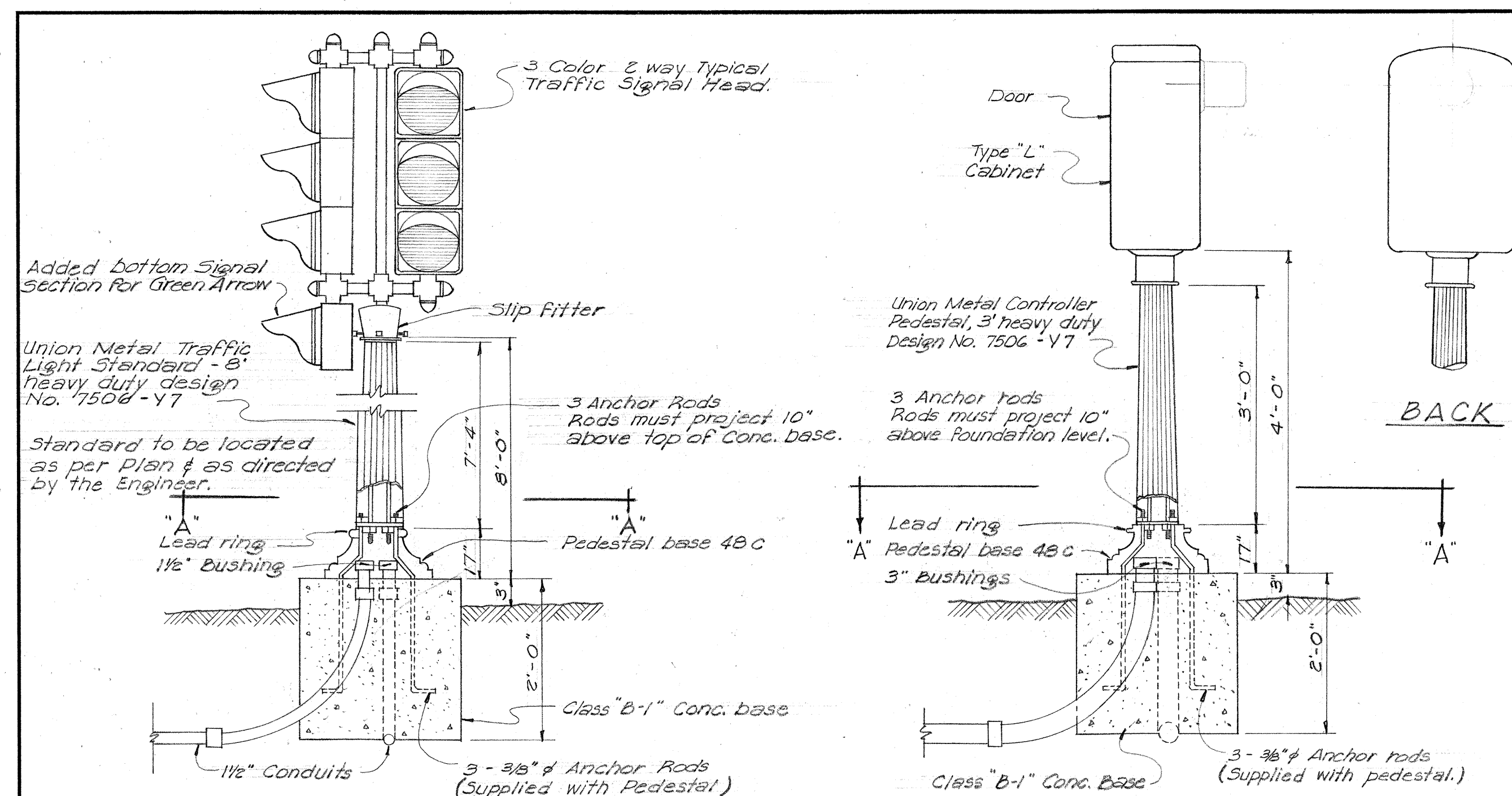
ELEVATION
