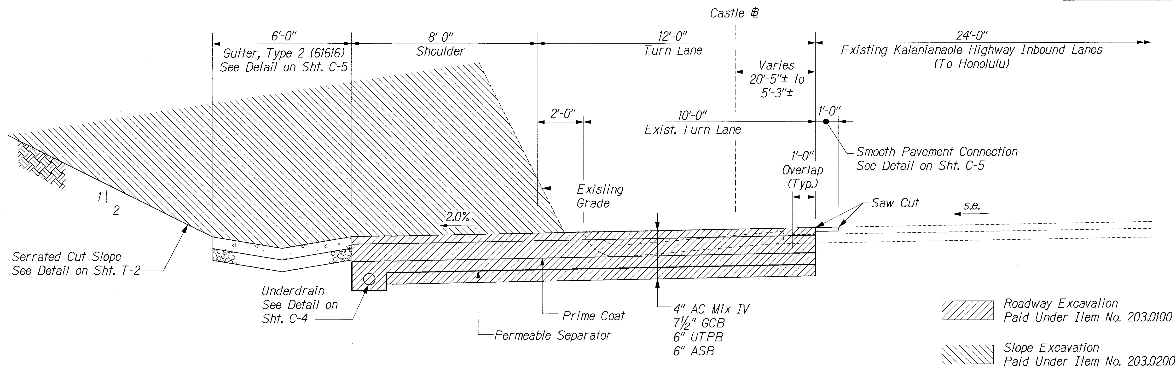
TYPICAL SECTION CASTLE # STA. 212+10 TO STA. 223+60 Scale: 1/2" = 1'-0"
