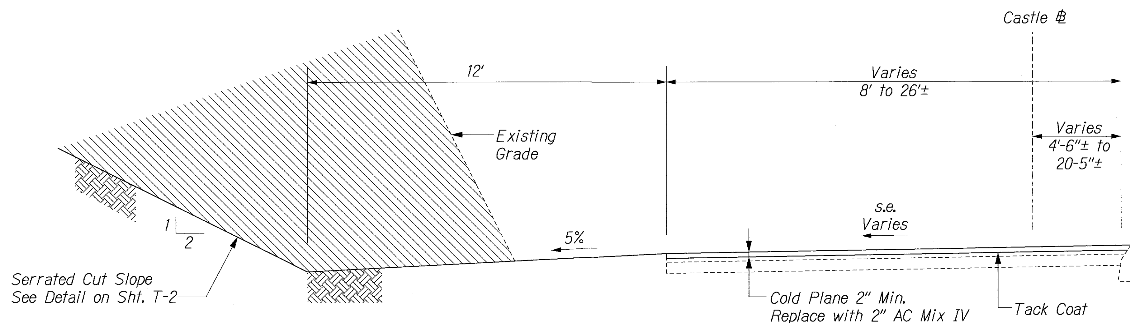
TYPICAL SECTION CASTLE # STA. 208+45 TO STA. 212+10 Scale: 1/2" = 1'-0"
