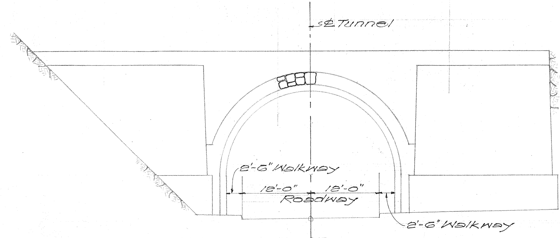
PORTAL 1 Scale: 1" = 10'-0"
