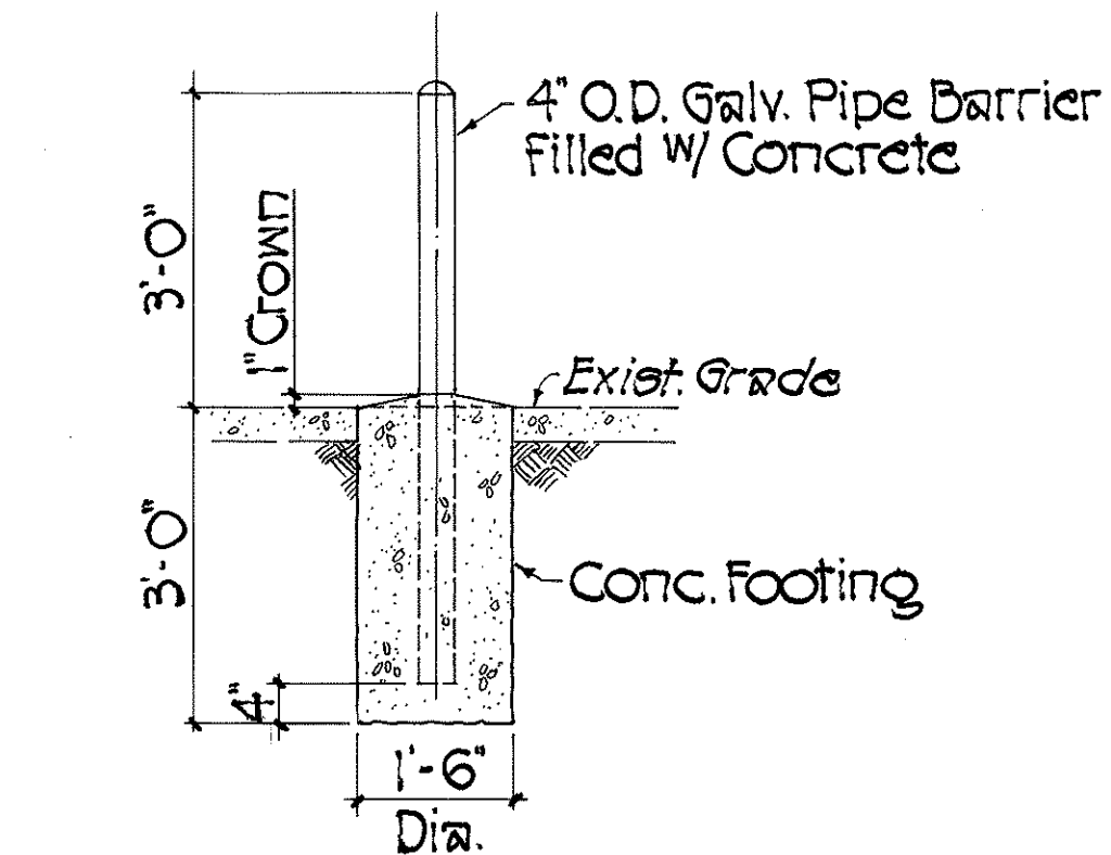
CONTROLLER BARRIER Scale: 1/2" = 1'-0"
