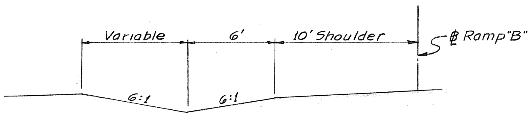
SECTION A-A
