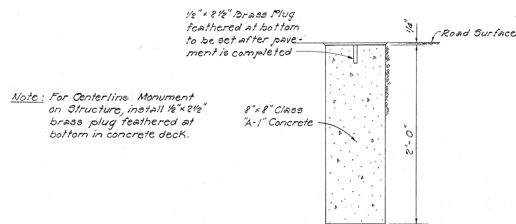
CENTERLINE MONUMENT Scale: 1 1/2" = 1'-0"
