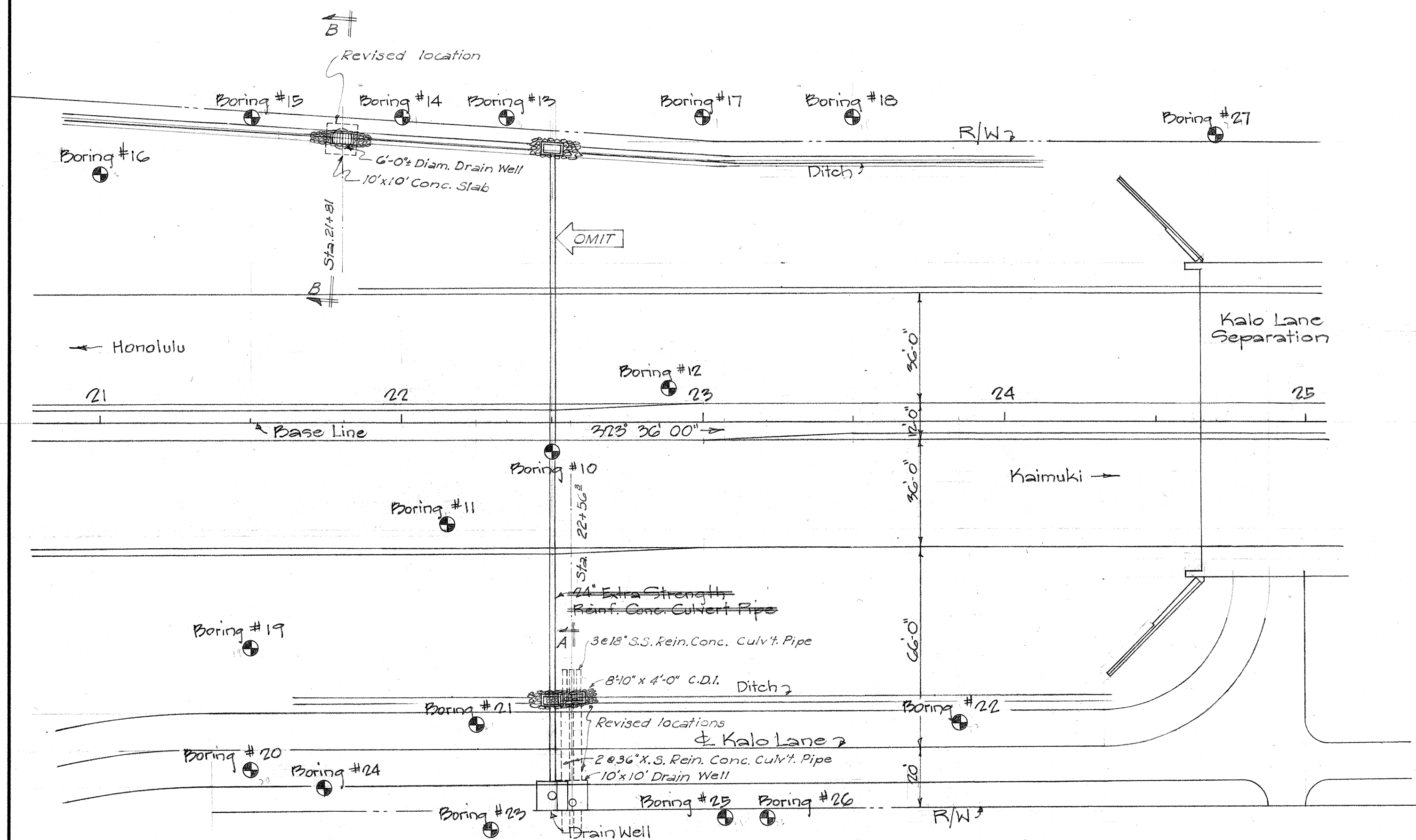
PLAN Scale: 1" = 30'
