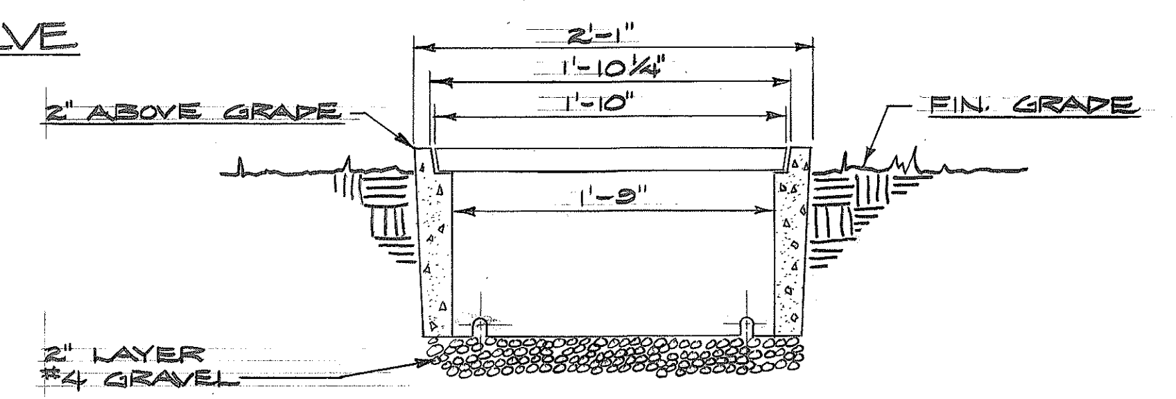
SECTION A-A
