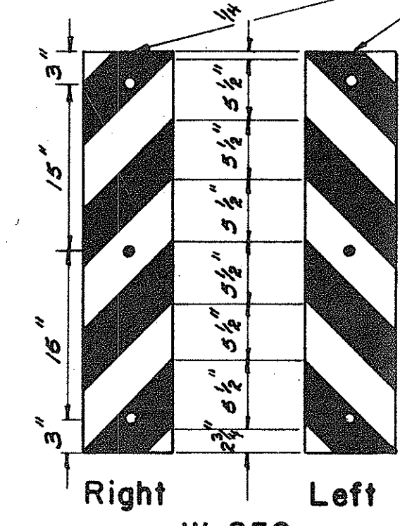
W-250 8" x 36"
