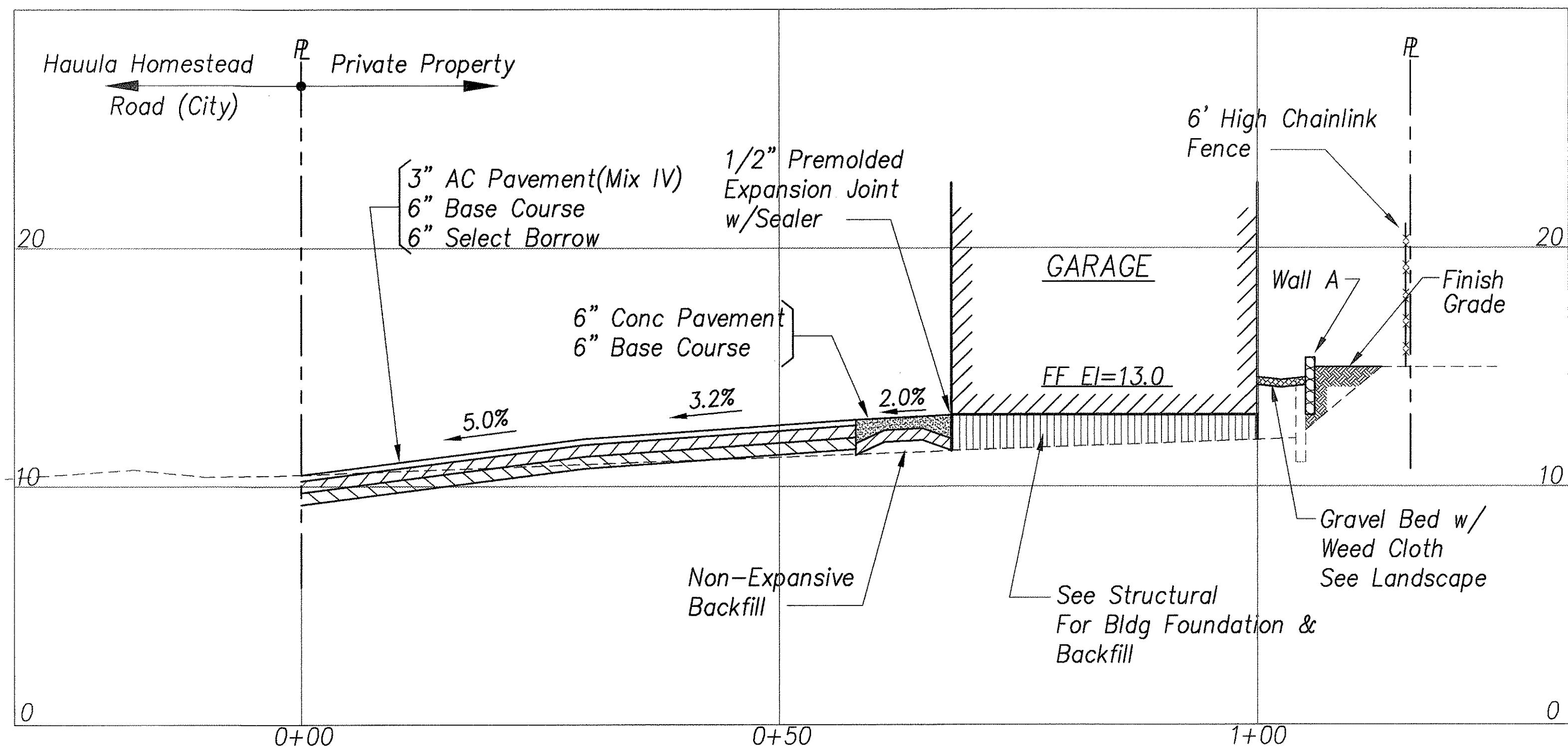
SECTION A-A/C2 SCALES: HORIZ 1"=10' VERT 1"=4'
