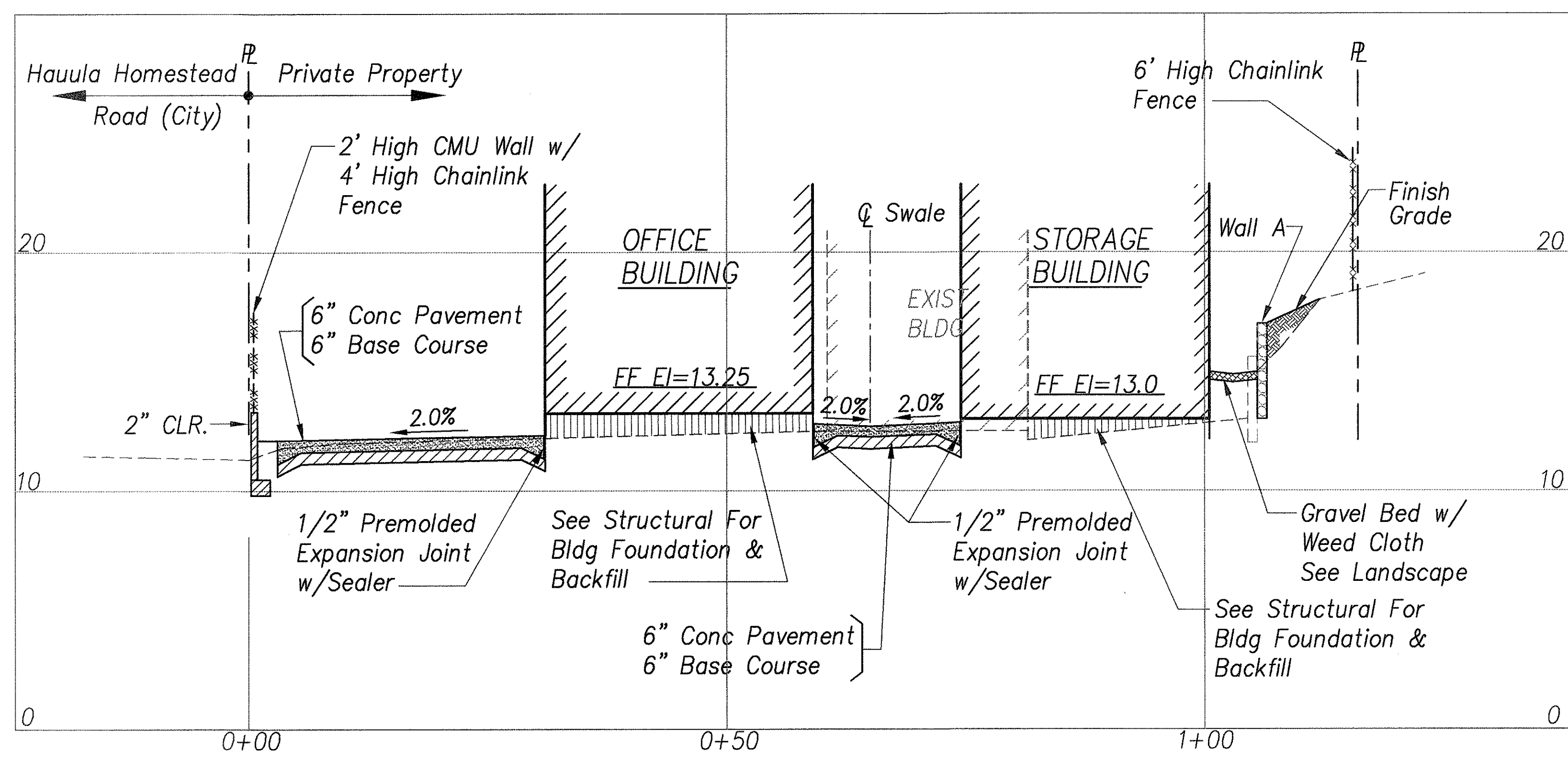
SECTION B-B/C2 SCALES: HORIZ 1"=10' VERT 1"=4'
