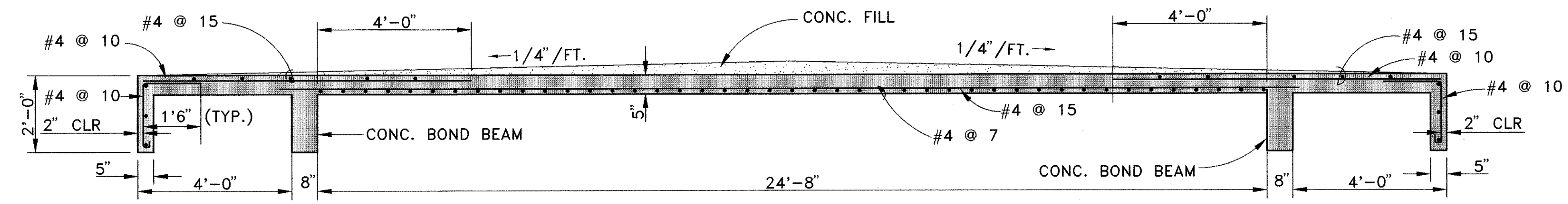
SECTION A SCALE: 1/2" = 1' 0"
