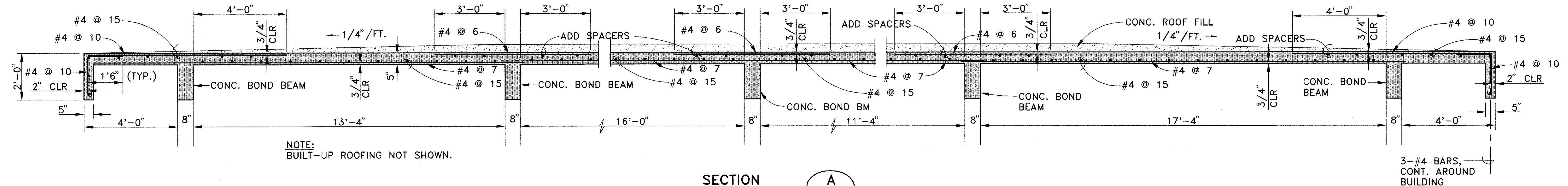
SECTION A SCALE: 1/2" = 1' 0"
