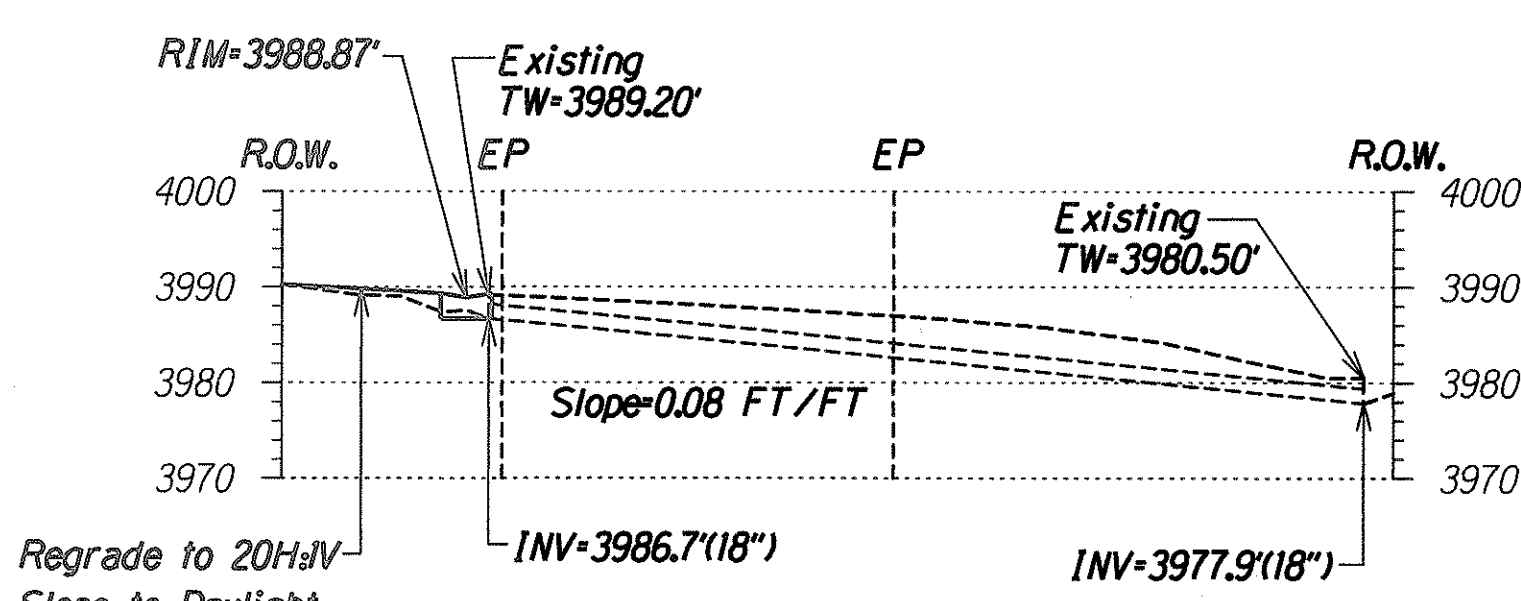
Profile IL-IL Scale: 1"=20'-0"
