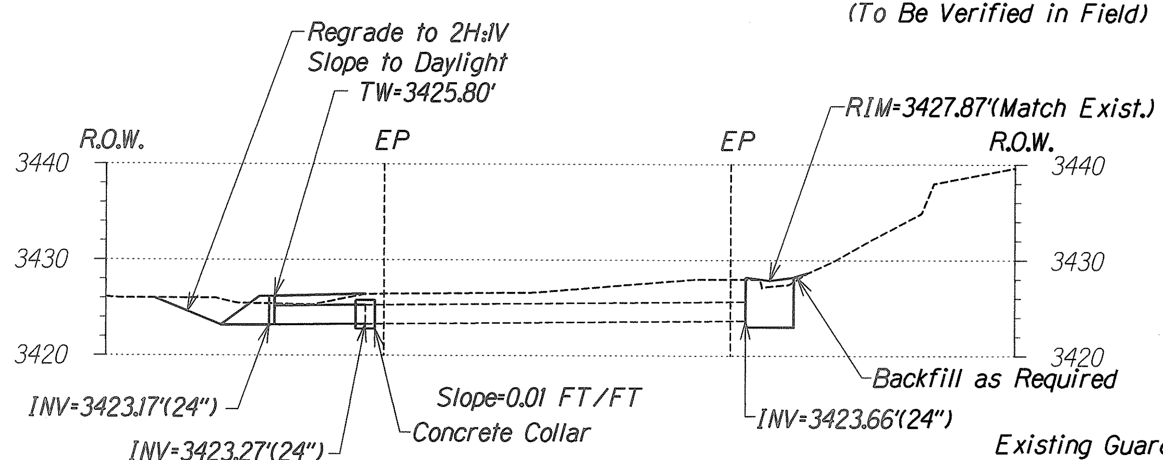
Profile A-A Scale: 1"=10'-0"
