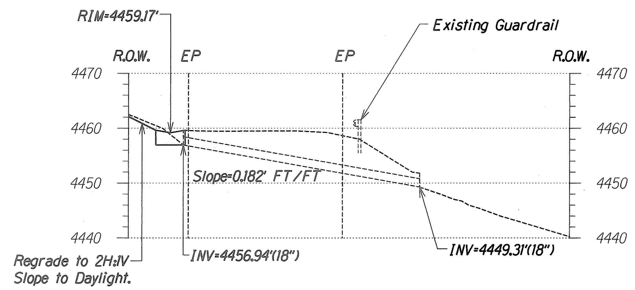
Profile S-S Scale: 1"=10'-0"
