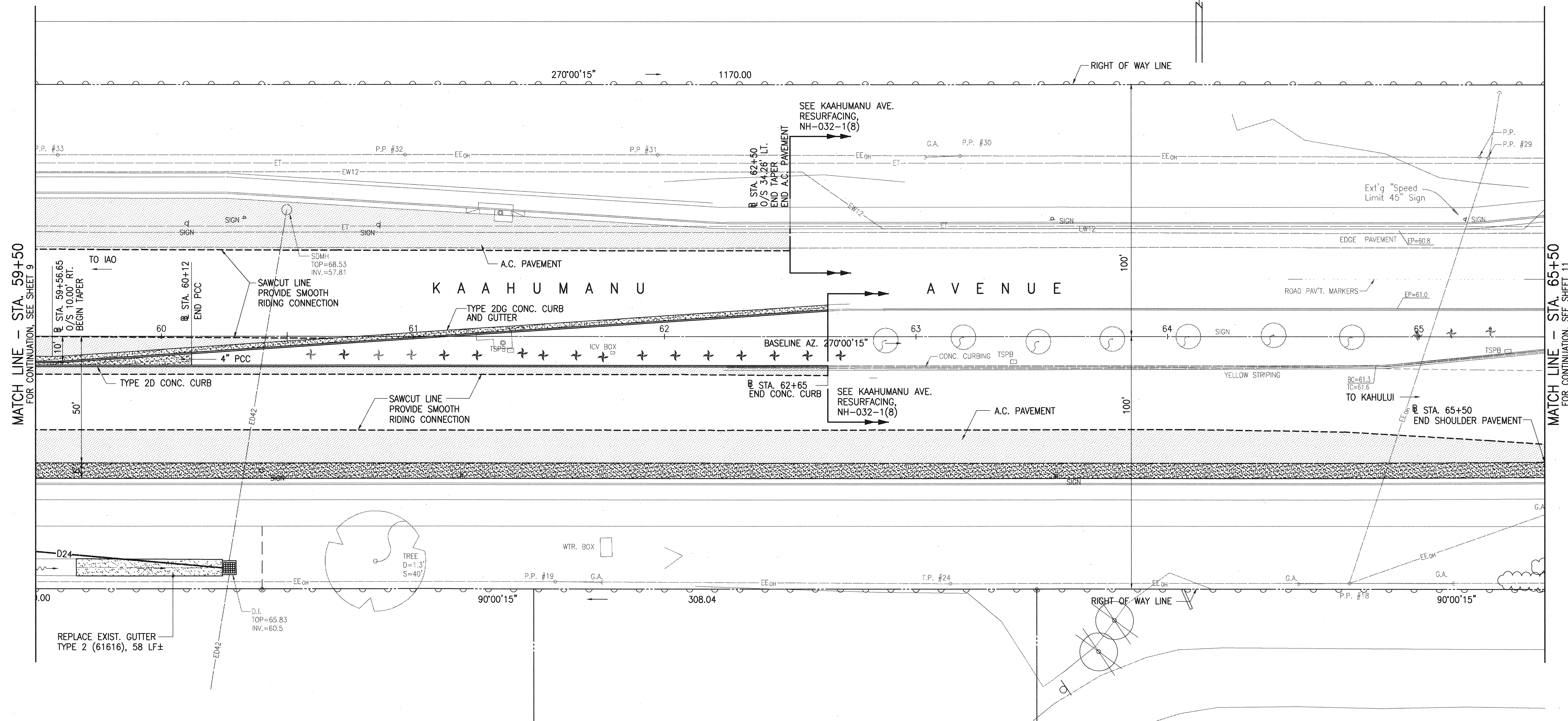
GEOMETRIC PLAN SCALE: 1"=20'
