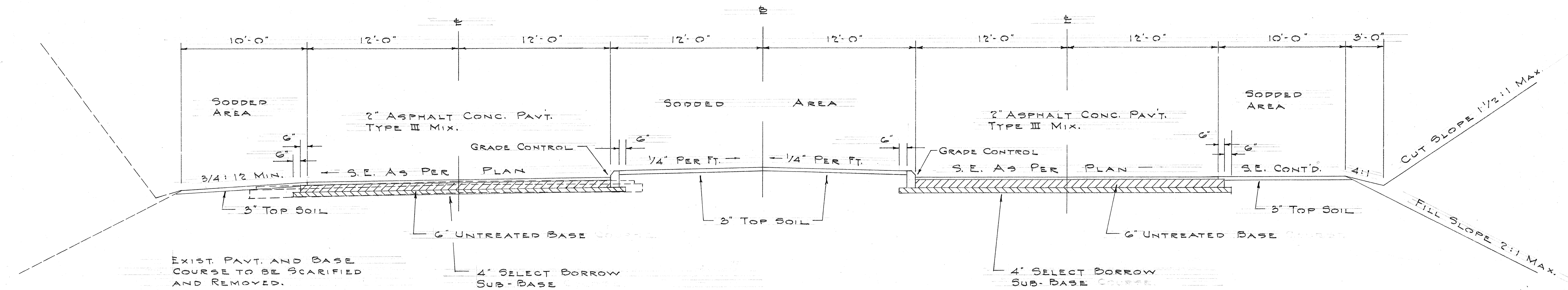
TYPICAL SECTION STA. 93+50 TO STA. 99+27.12 SCALE: 1/4" = 1'-0"
