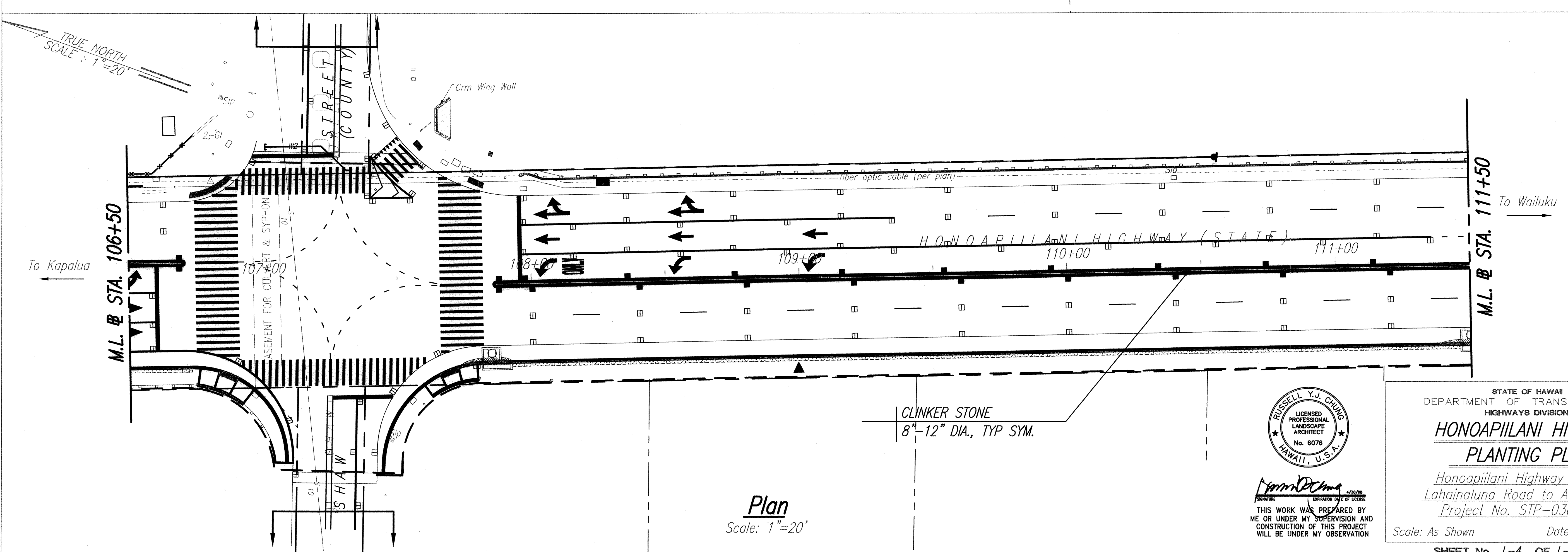
Plan Scale: 1"=20'
