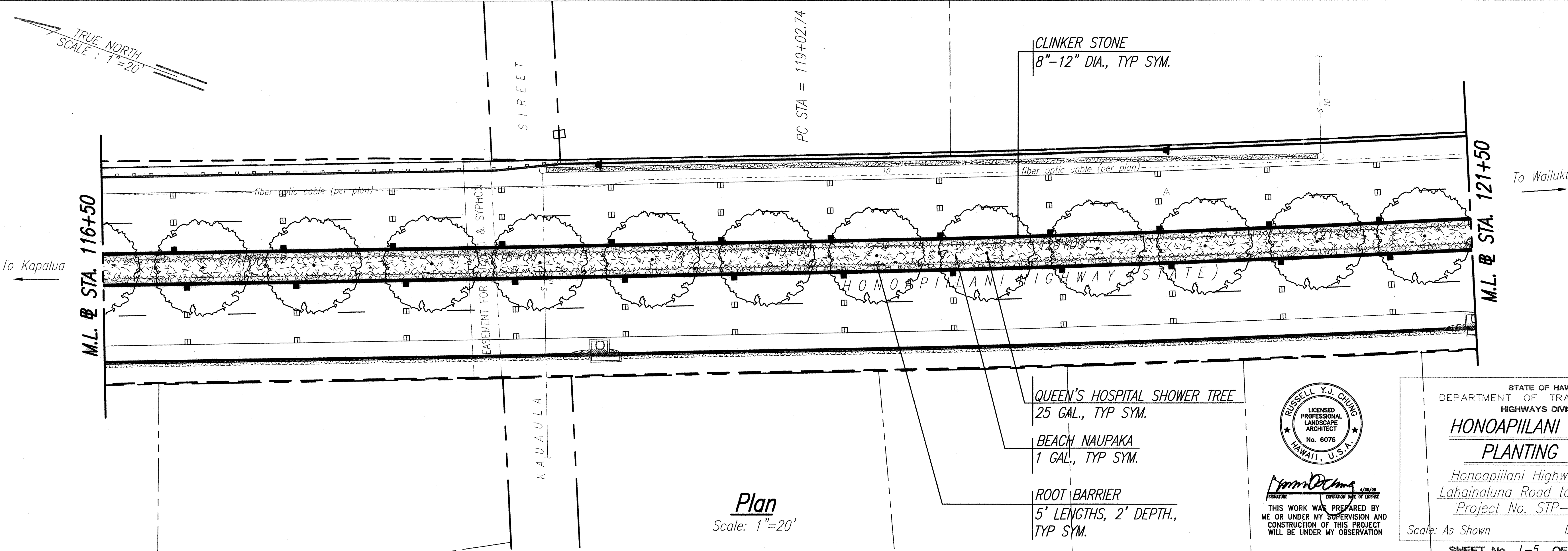
Plan Scale: 1"=20'
