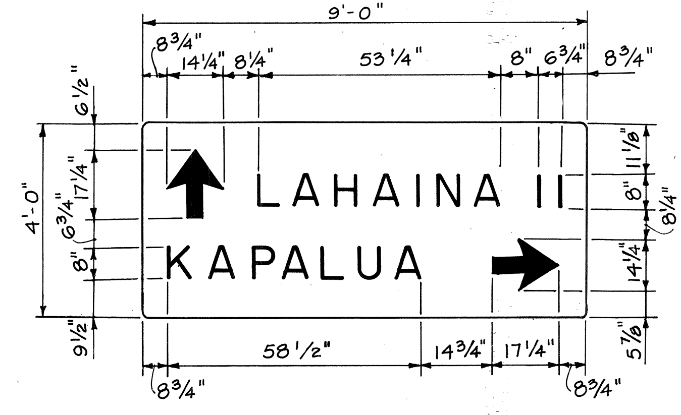
SIGN DIR-2 N.T.S.
