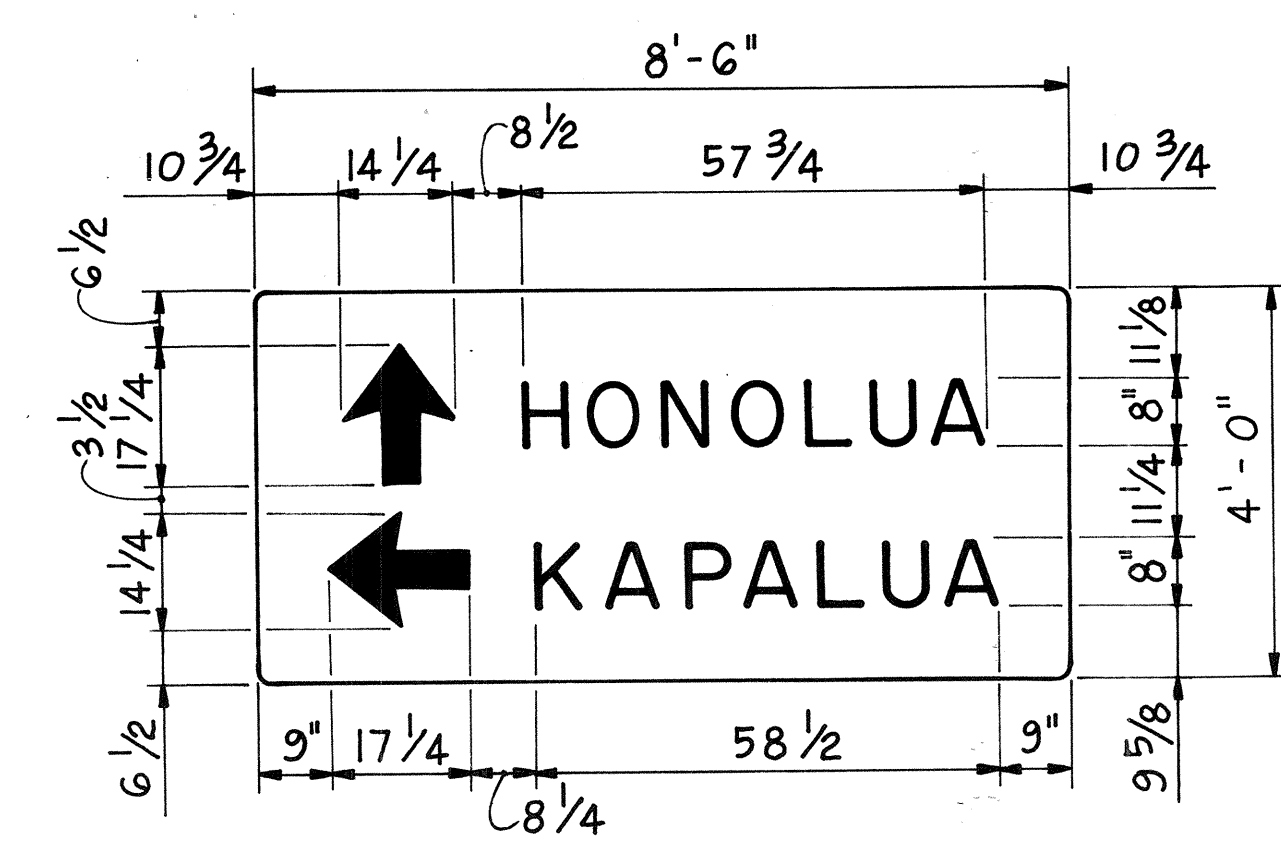
SIGN DIR-1 N.T.S.
