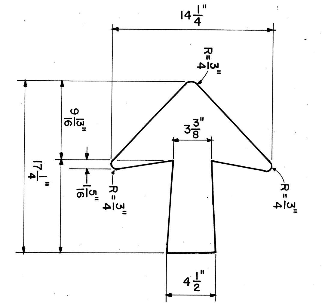
DIRECTION SIGN ARROW DETAIL N.T.S.
