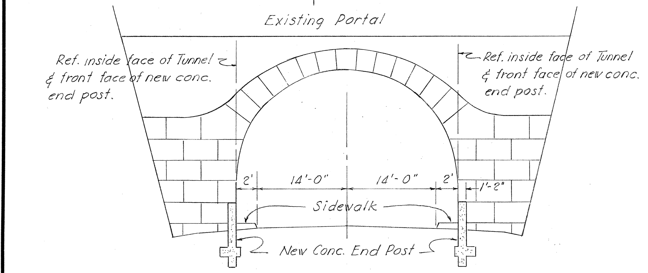
PORTAL ELEVATION Scale: 1/8" = 1'-0"
