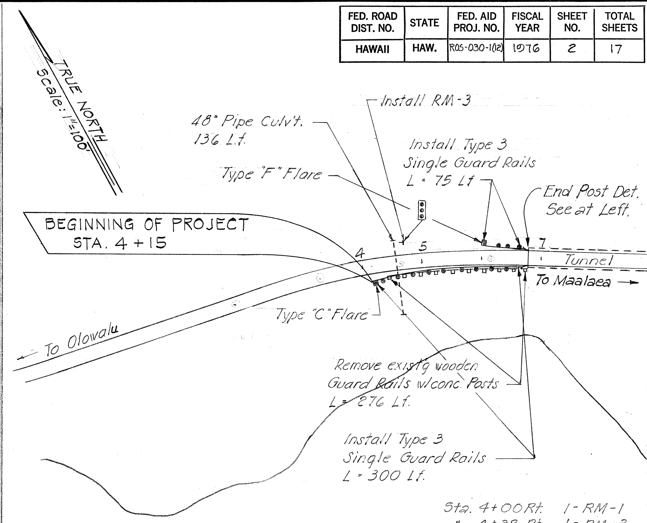
PLAN Scale: 1" = 100'
