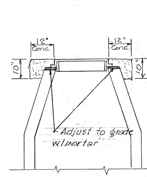
ADJUSTED MANHOLE Scale: 1/2" = 1'-0"
