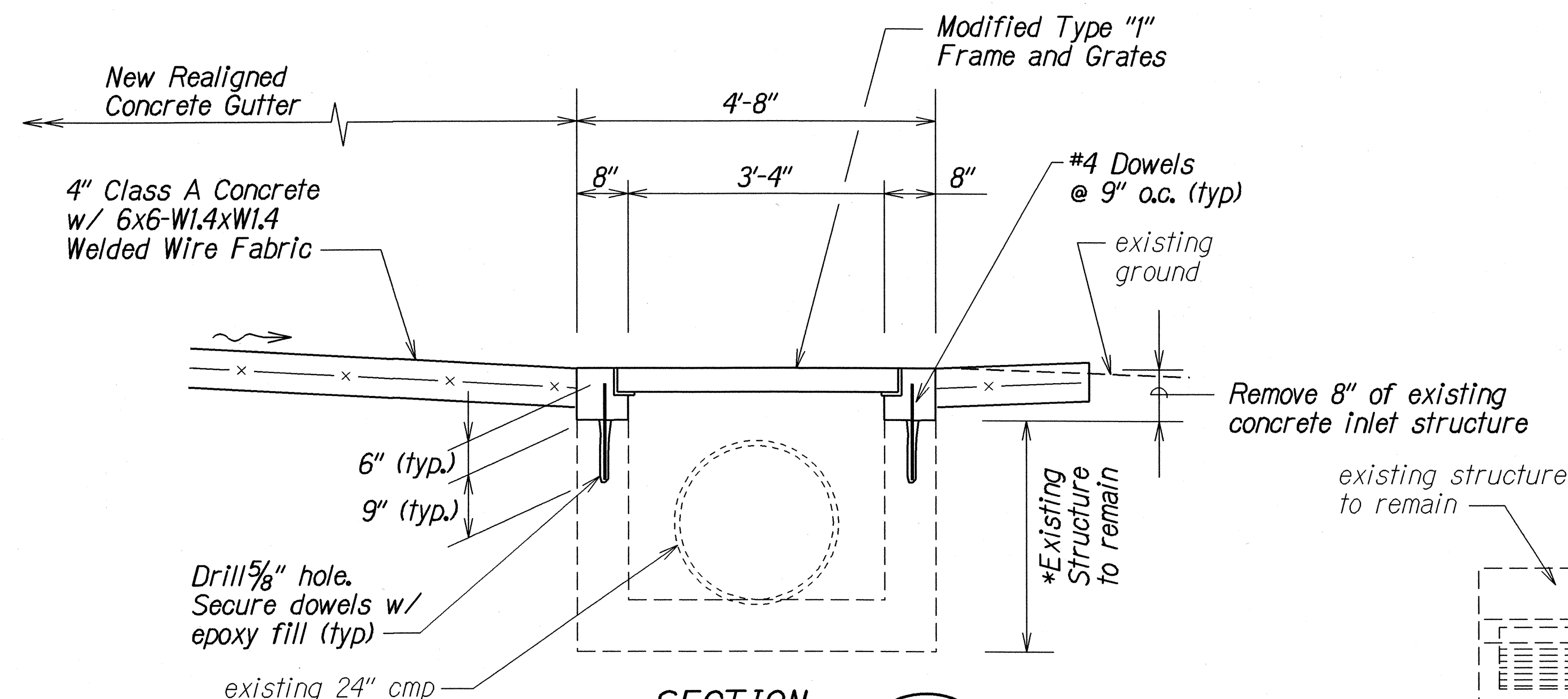
SECTION Scale: 3/4"=1'-0"
