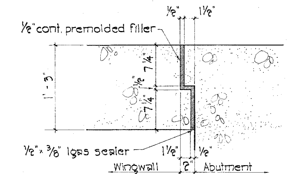
DETAIL 2 N.T.S.
