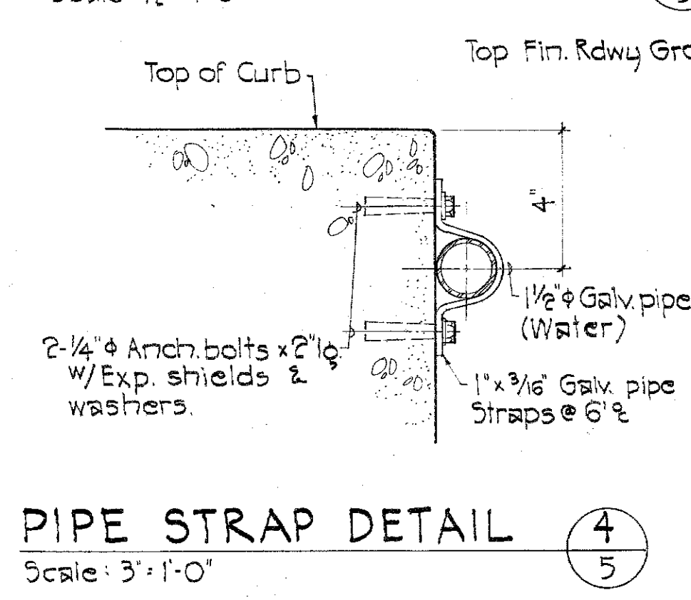
PIPE STRAP DETAIL Scale: 3" = 1'-0"
