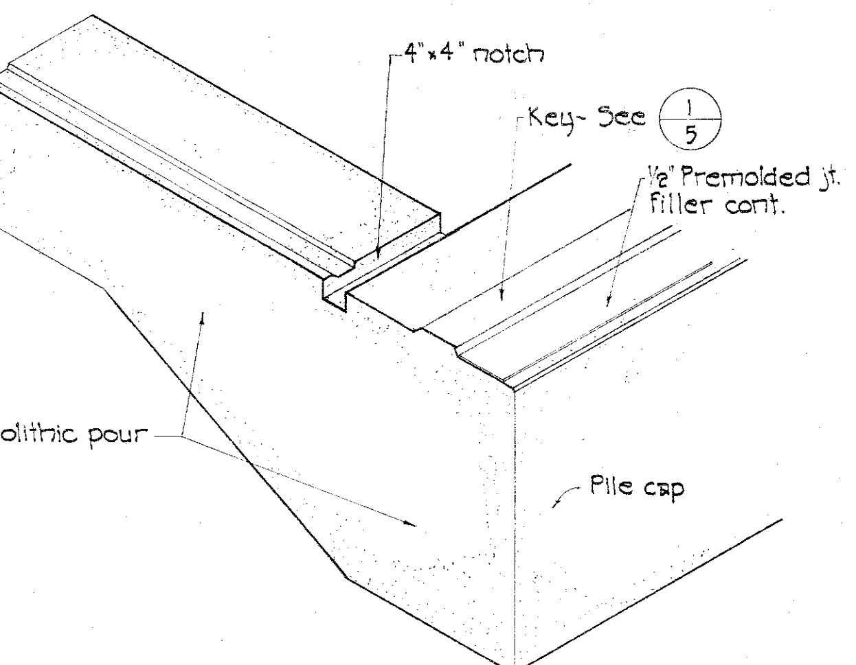
END POST GROOVE DETAIL Scale: 3" = 1'-0"
