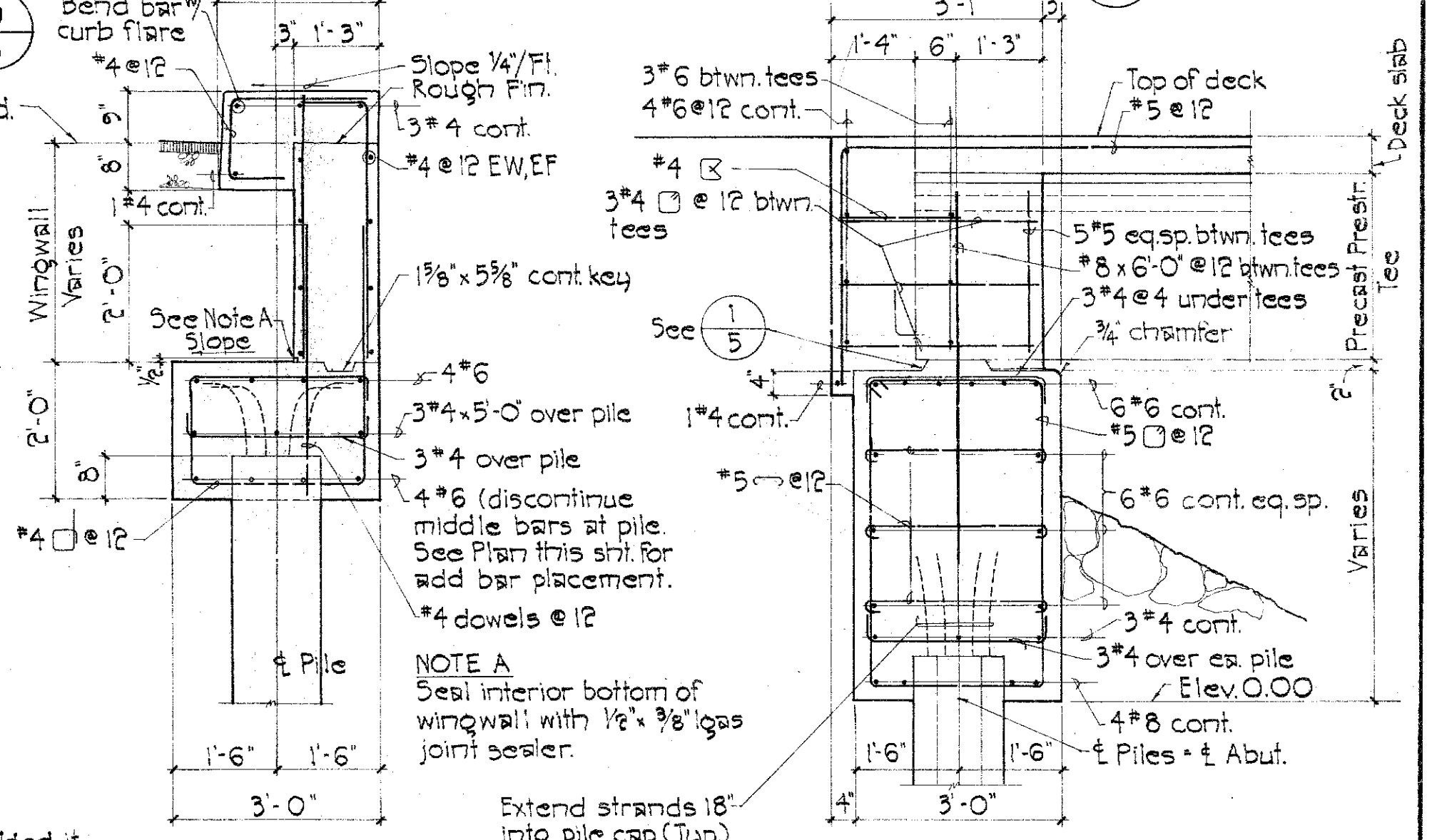
SECTION ELEVATION Scale: 1/2" = 1'-0"
