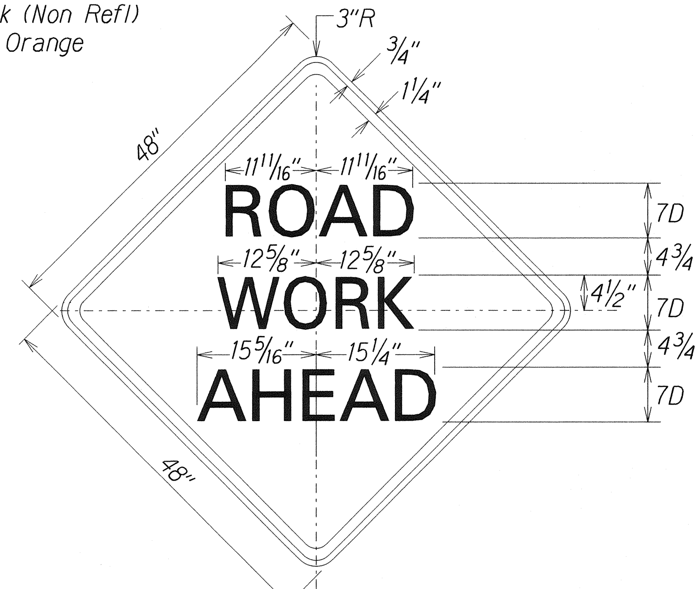
CW20-1A(d) Scale: 1" = 1'-0"
