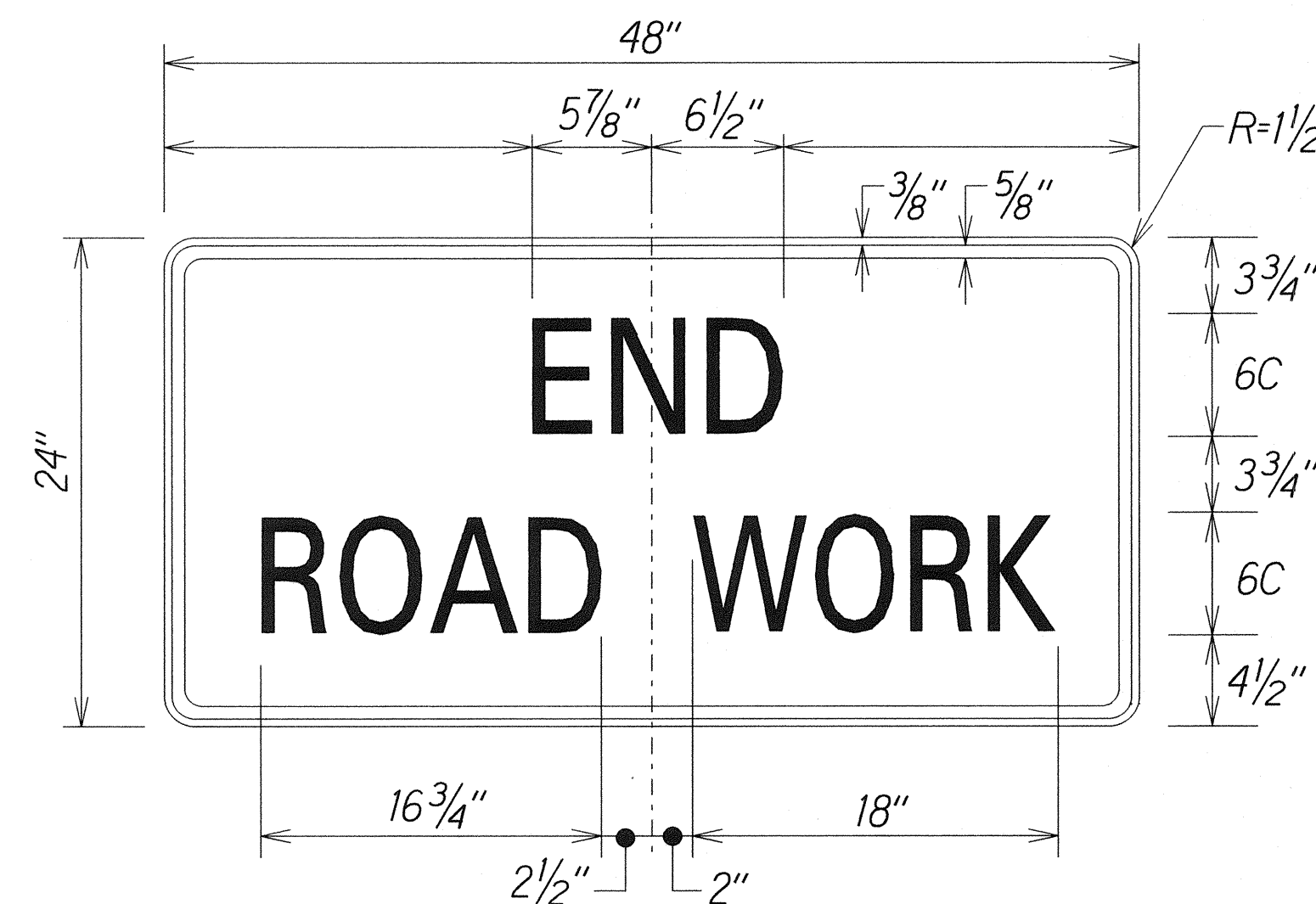
CG20-2A Scale: 1 1/2" = 1'-0"
