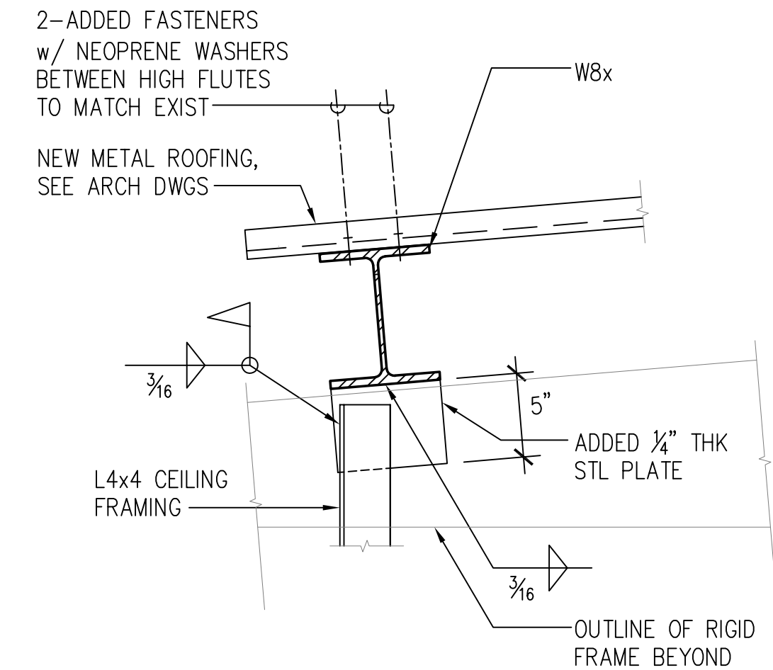
1 S-7 DETAIL SCALE: 1 1/2"=1'-0"
