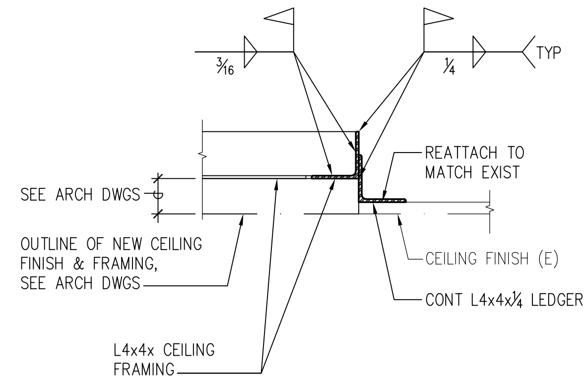
5 S-7 SECTION SCALE: 1 1/2"=1'-0"
