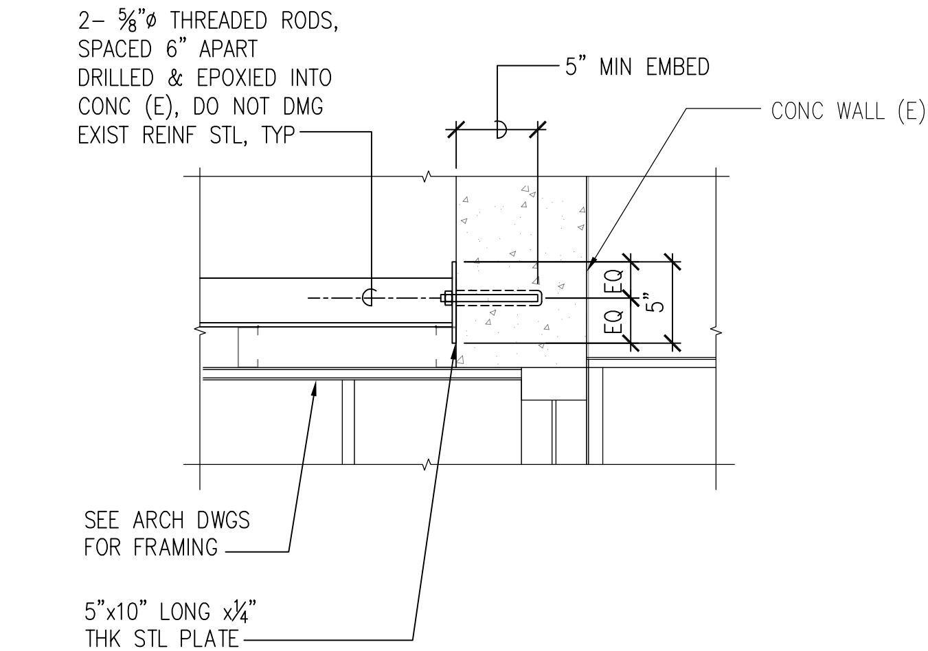
3 S-7 DETAIL SCALE: 1 1/2"=1'-0"
