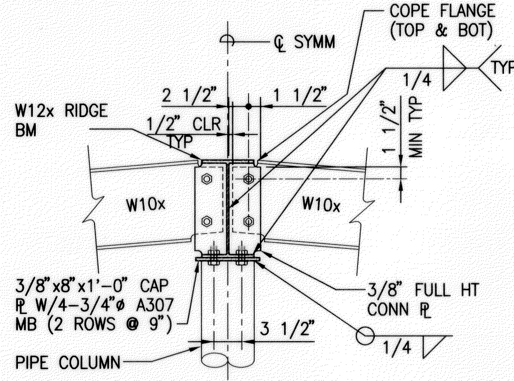
2 SECTION S7.1 SCALE: 1"=1'-0"
