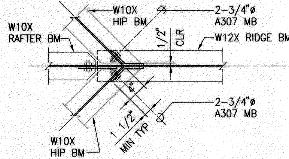
5B SECTION S7.1 SCALE: 1"=1'-0"
