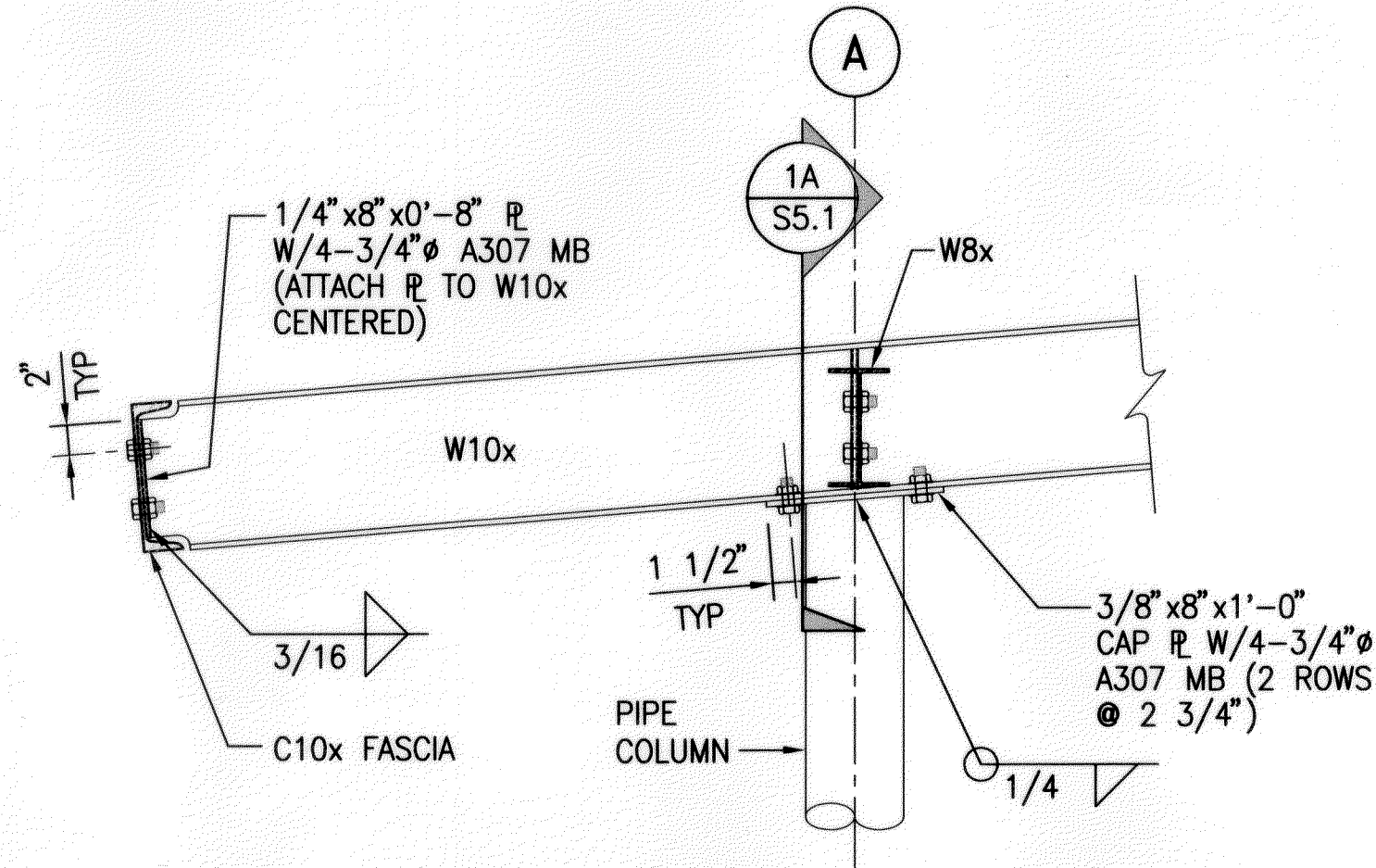
1 SECTION S7.1 SCALE: 1"=1'-0"
