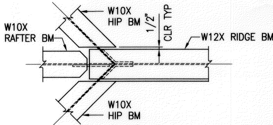
5A SECTION S7.1 SCALE: 1"=1'-0"
