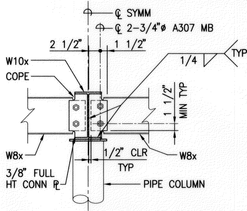
1A SECTION S7.1 SCALE: 1"=1'-0"
