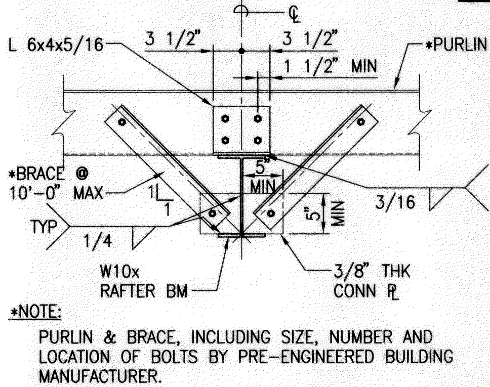
3 SECTION S7.1 SCALE: 1"=1'-0"
