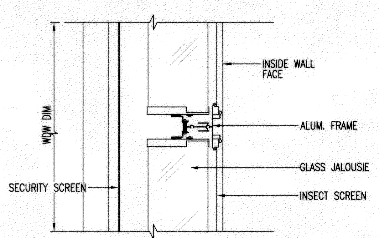
13 MULLION A5.6 SCALE: 3"=1'-0"
