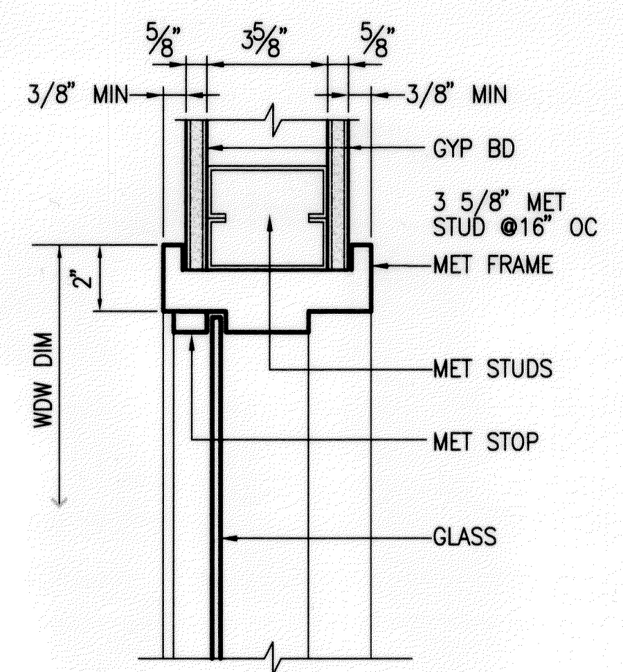
7 HEAD/JAMB A5.6 SCALE: 3"=1'-0"
