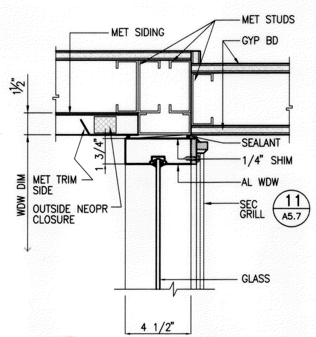
4 JAMB A5.6 SCALE: 3"=1'-0"
