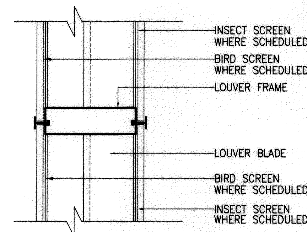
4 MULLION A5.7 SCALE: 3"=1'-0"
