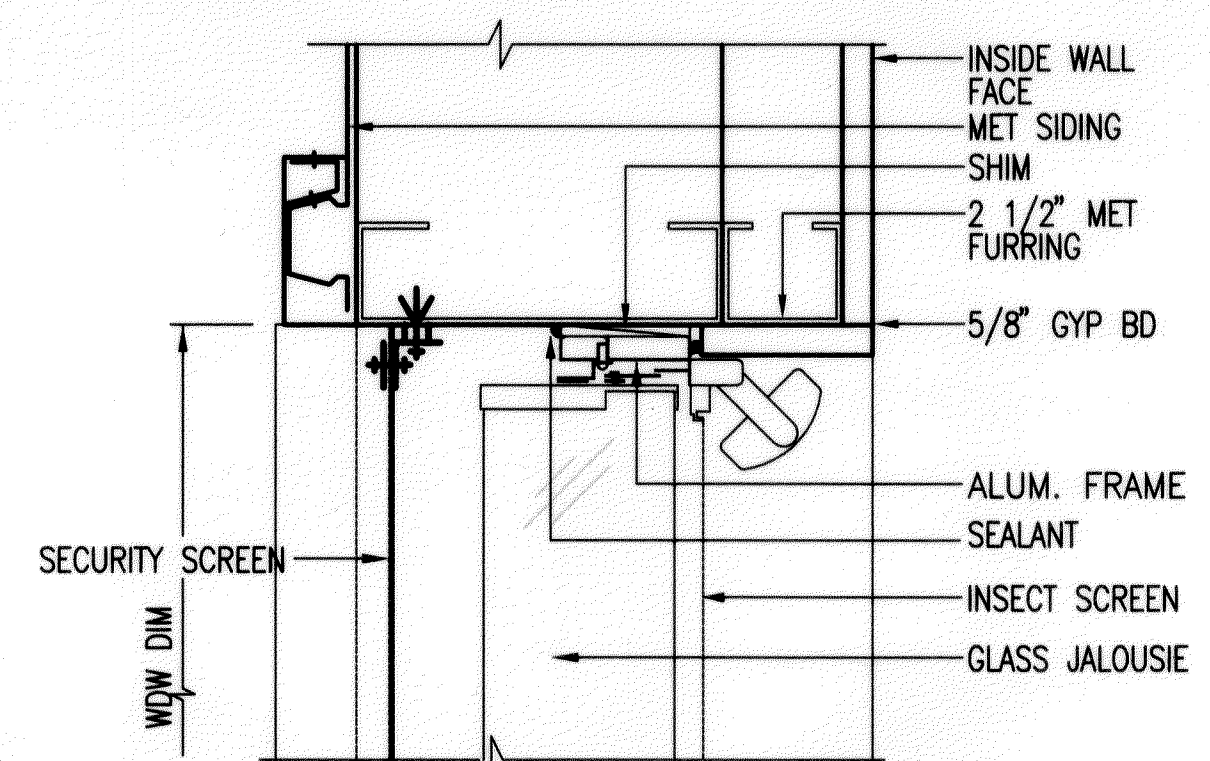
8 JAMB A5.6 SCALE: 3"=1'-0"
