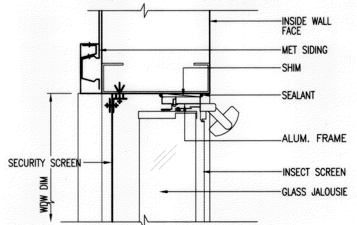
12 JAMB A5.6 SCALE: 3"=1'-0"
