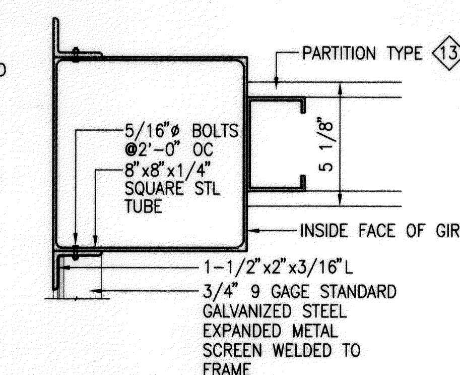
10 JAMB @ PARTITION A5.7 SCALE: 3"=1'-0"
