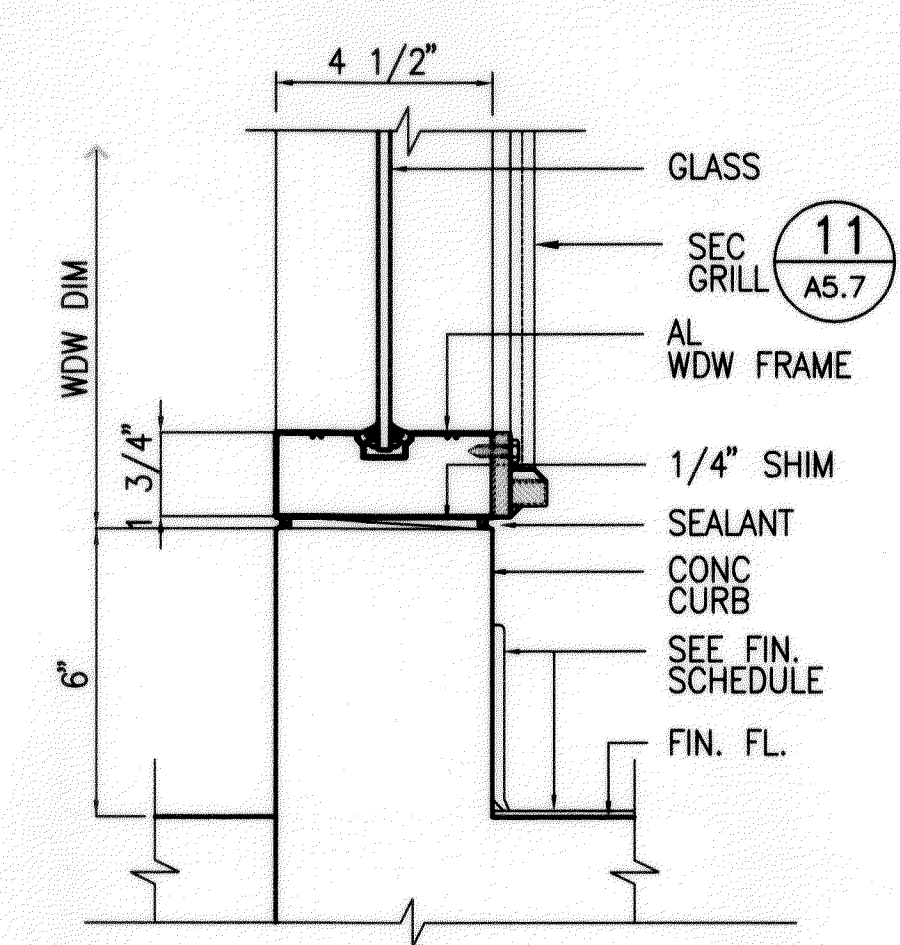
3 SILL A5.6 SCALE: 3"=1'-0"
