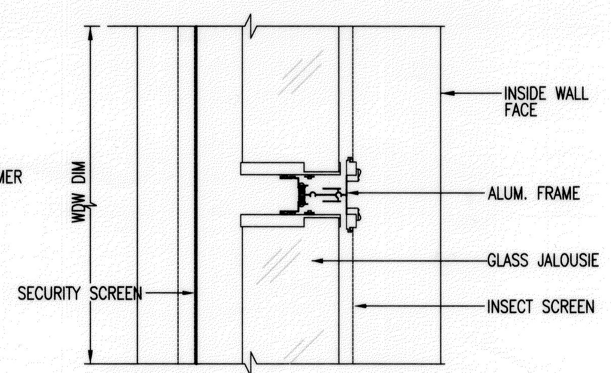
9 MULLION A5.6 SCALE: 3"=1'-0"
