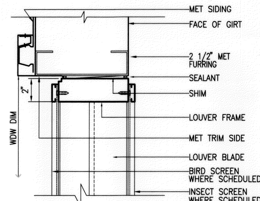
3 JAMB A5.7 SCALE: 3"=1'-0"
