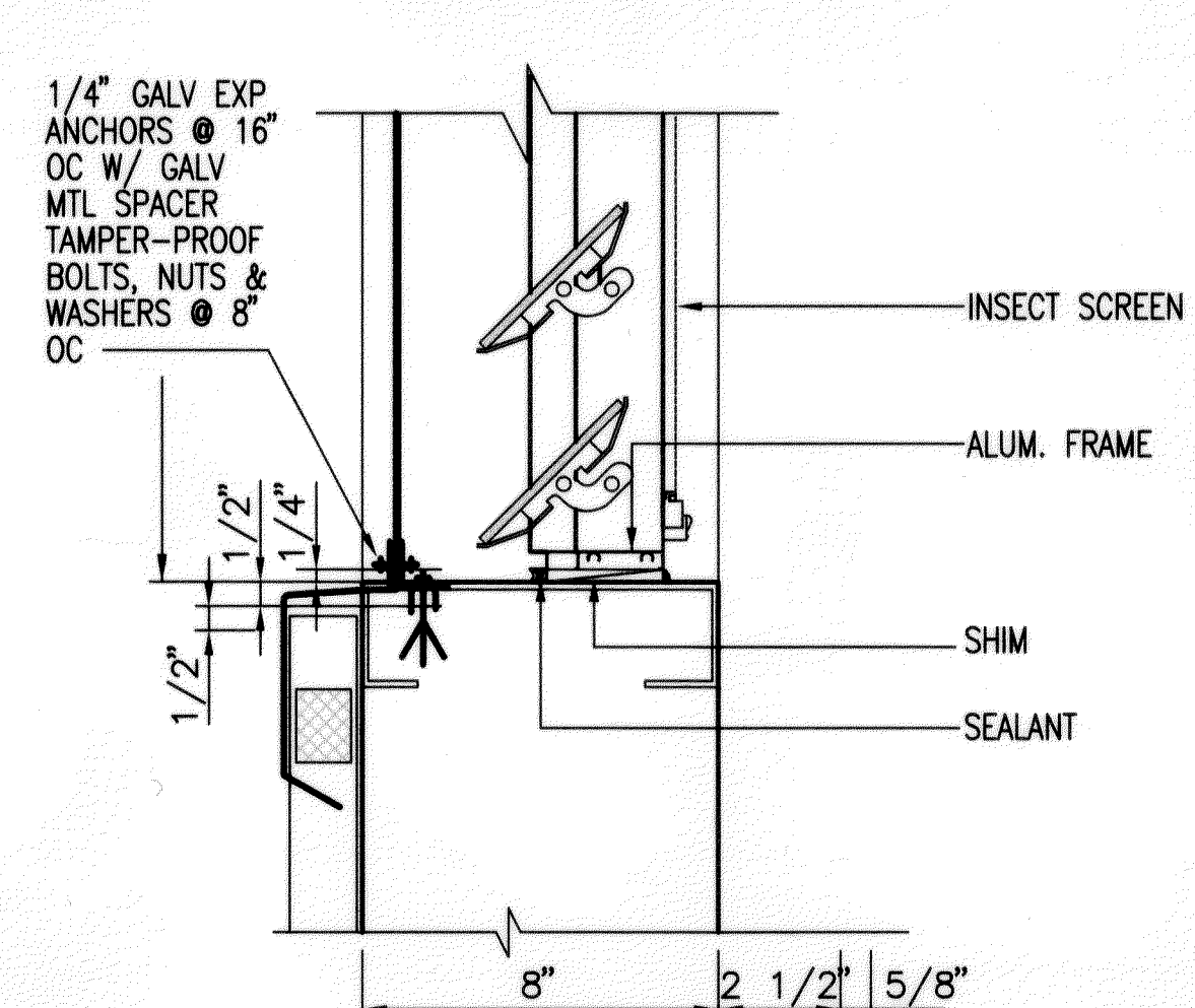
11 SILL A5.6 SCALE: 3"=1'-0"
