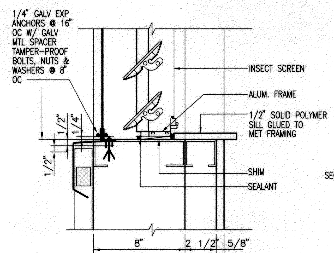
6 SILL A5.6 SCALE: 3"=1'-0"
