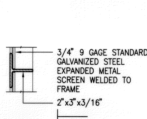
6 MULLION A5.7 SCALE: 3"=1'-0"
