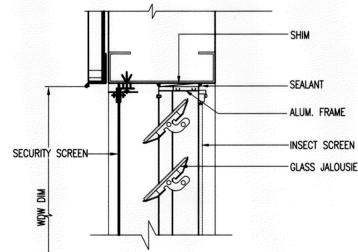
10 HEAD A5.6 SCALE: 3"=1'-0"
