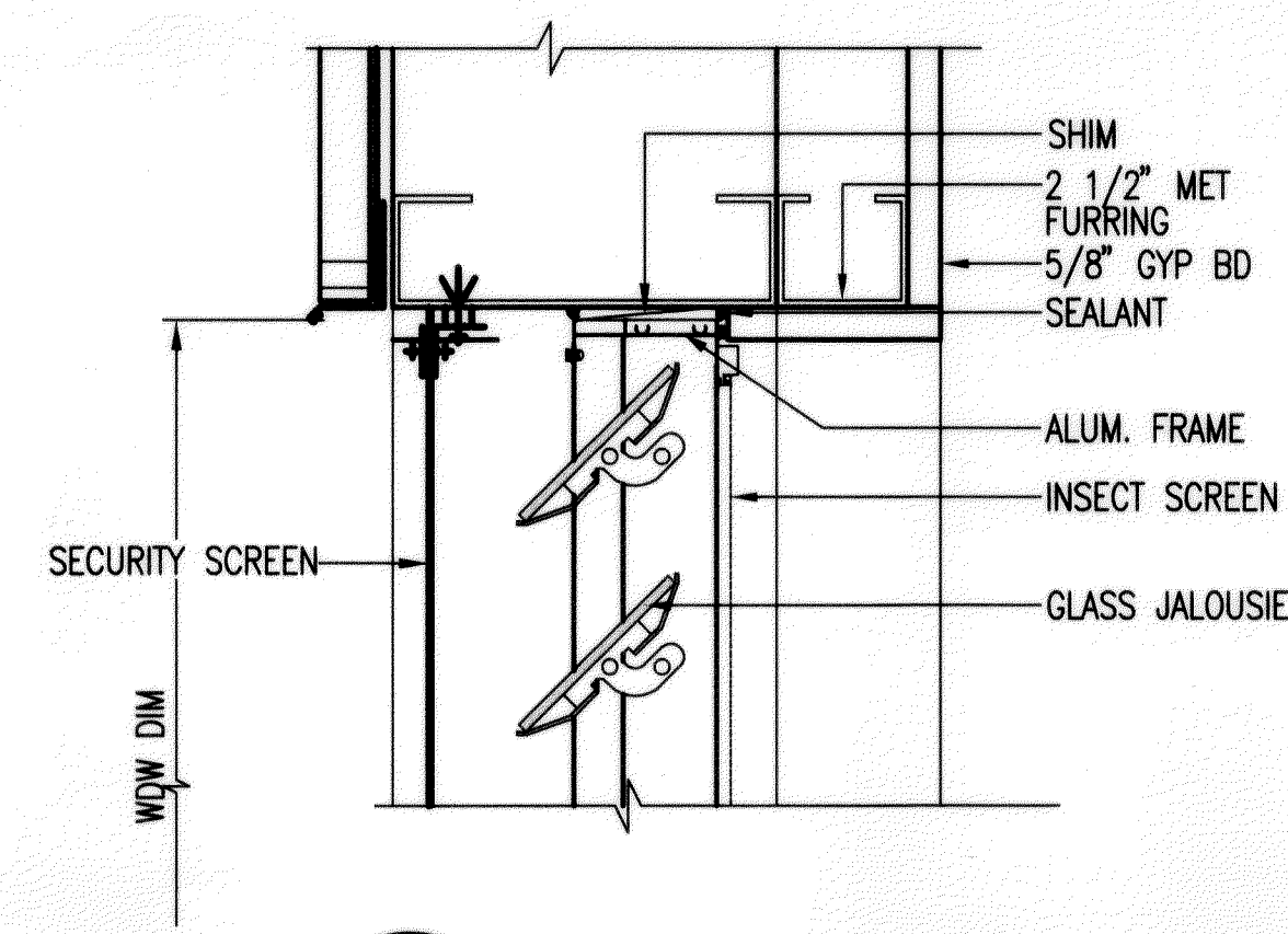
5 HEAD A5.6 SCALE: 3"=1'-0"
