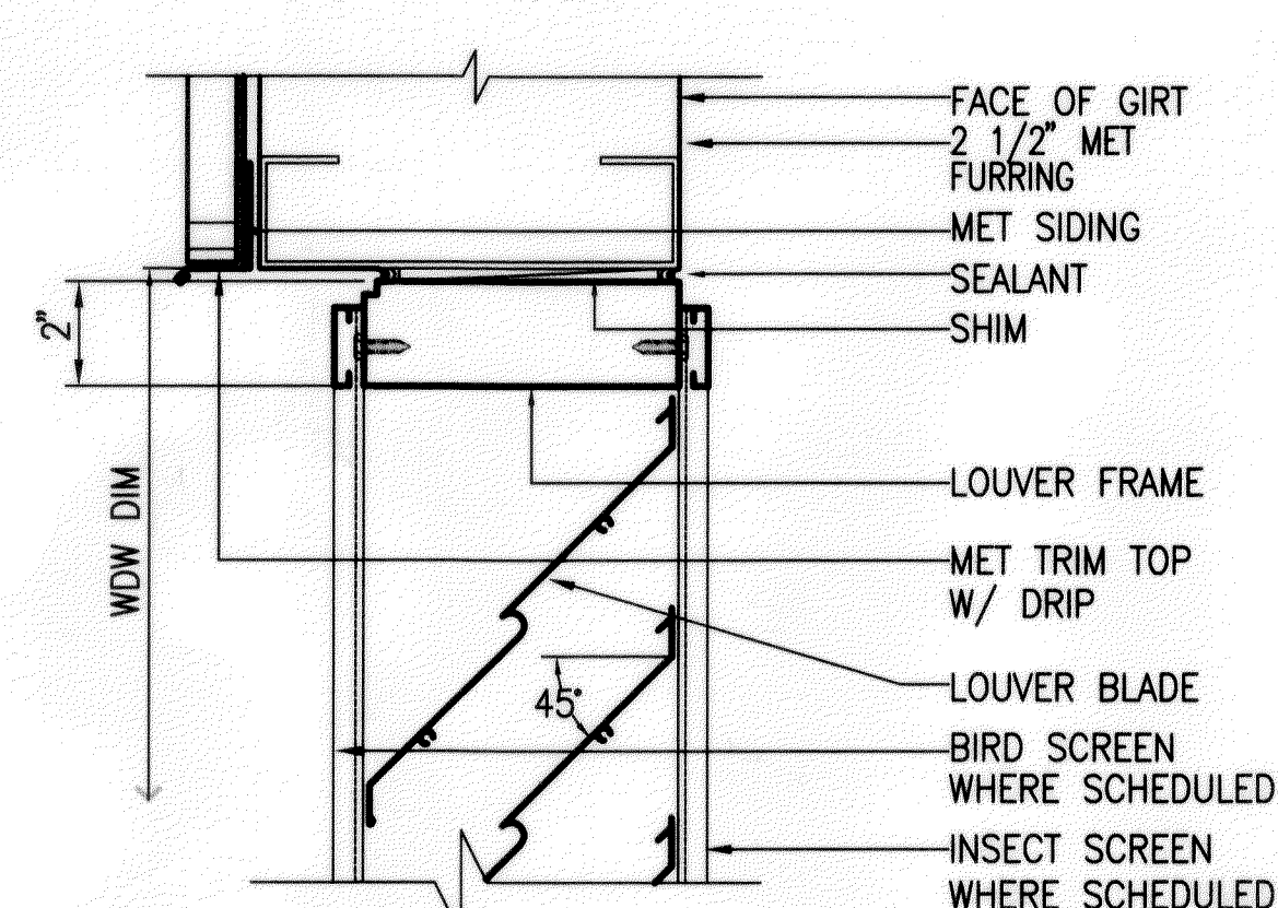
1 HEAD A5.7 SCALE: 3"=1'-0"
