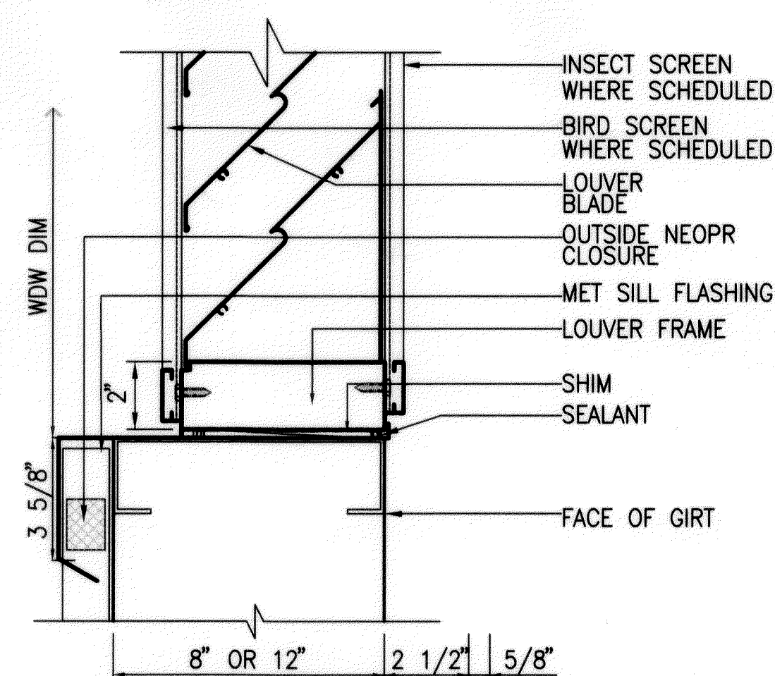
2 SILL A5.7 SCALE: 3"=1'-0"
