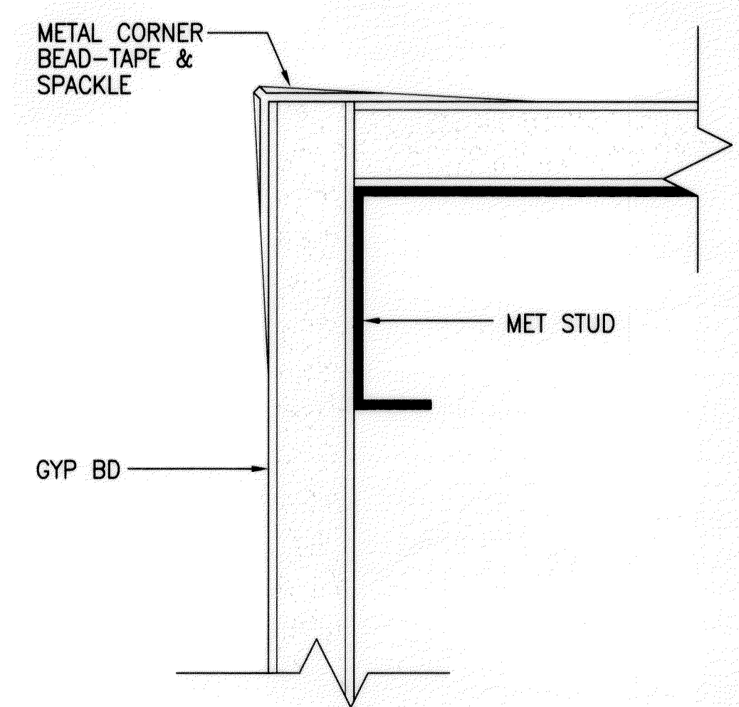
7 TYP DRYWALL CORNER DETAIL A7.3 SCALE: 6"=1'-0"
