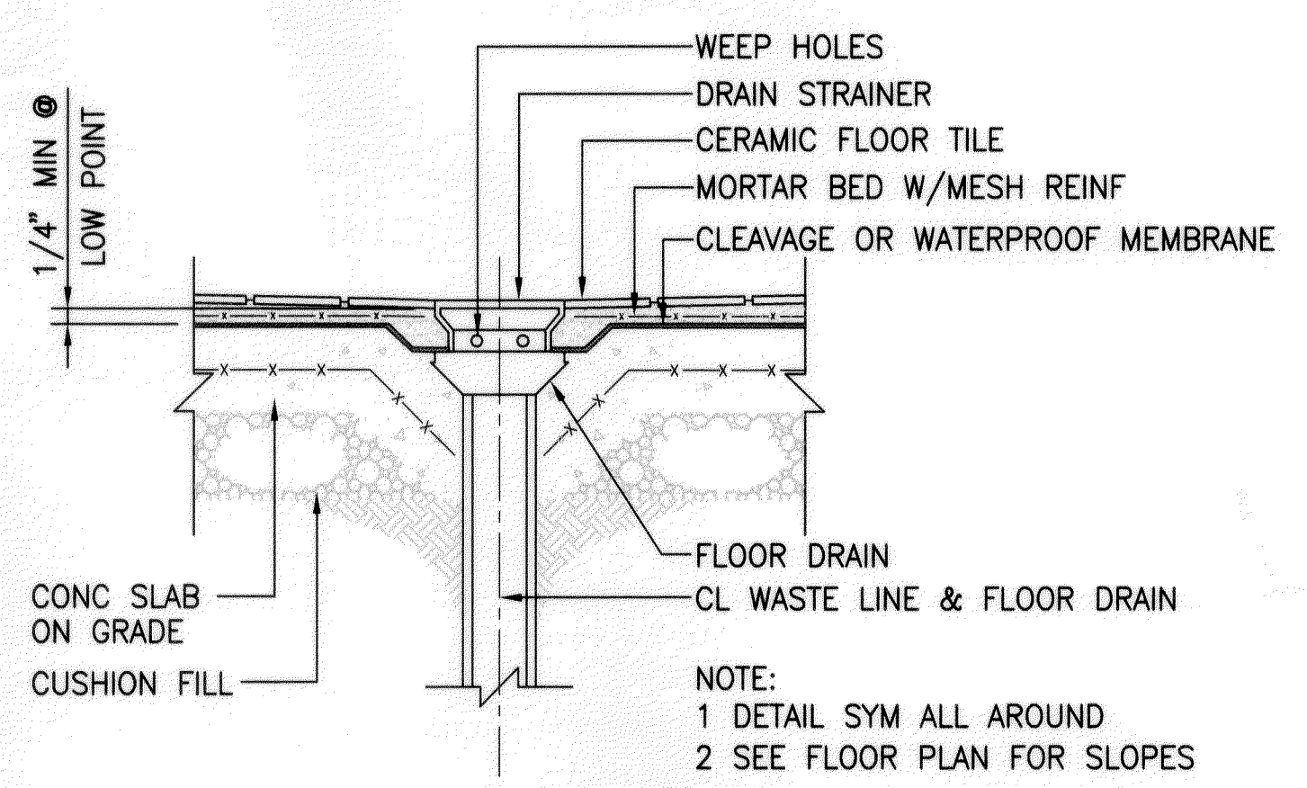
6 TYP FLOOR DRAIN DETAIL A7.3 SCALE: 1 1/2"=1'-0"
