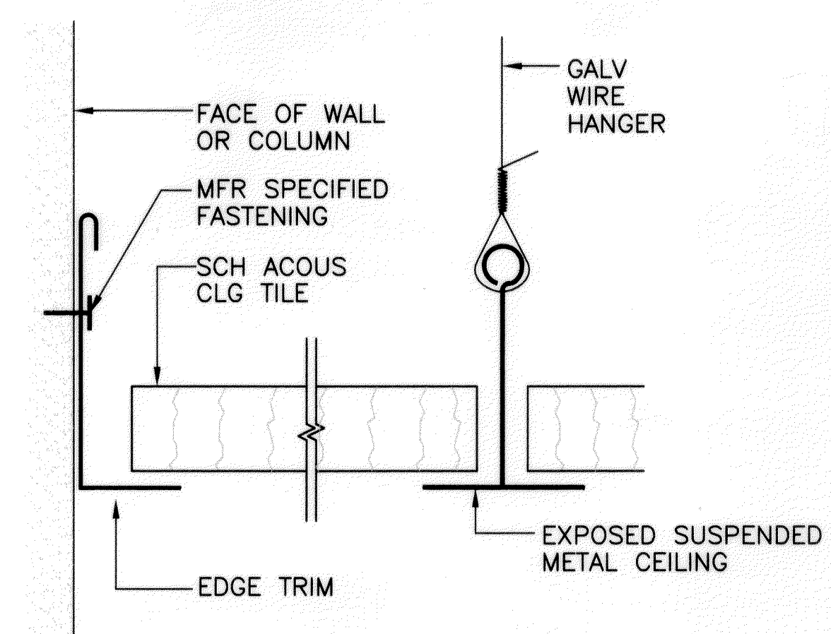
9 SUSP ACOUSTIC CEILING TILE A7.3 SCALE: 6"=1'-0"
