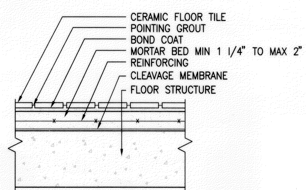
TCA DESIGN F111
