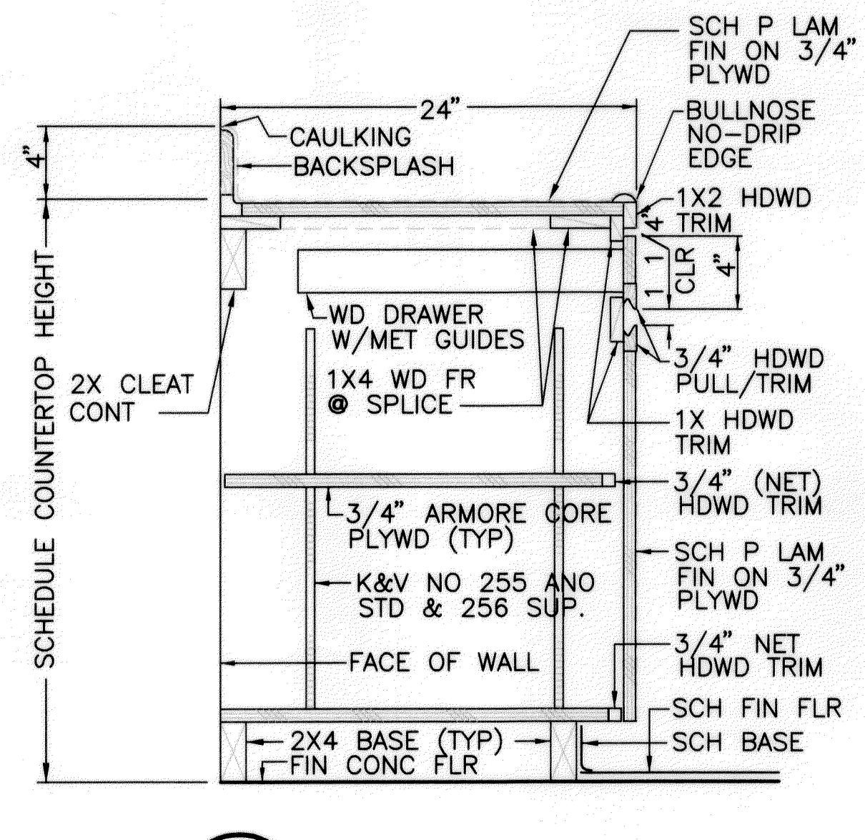
2 BASE CAB A7.4 SCALE: 1 1/2"=1'-0"
