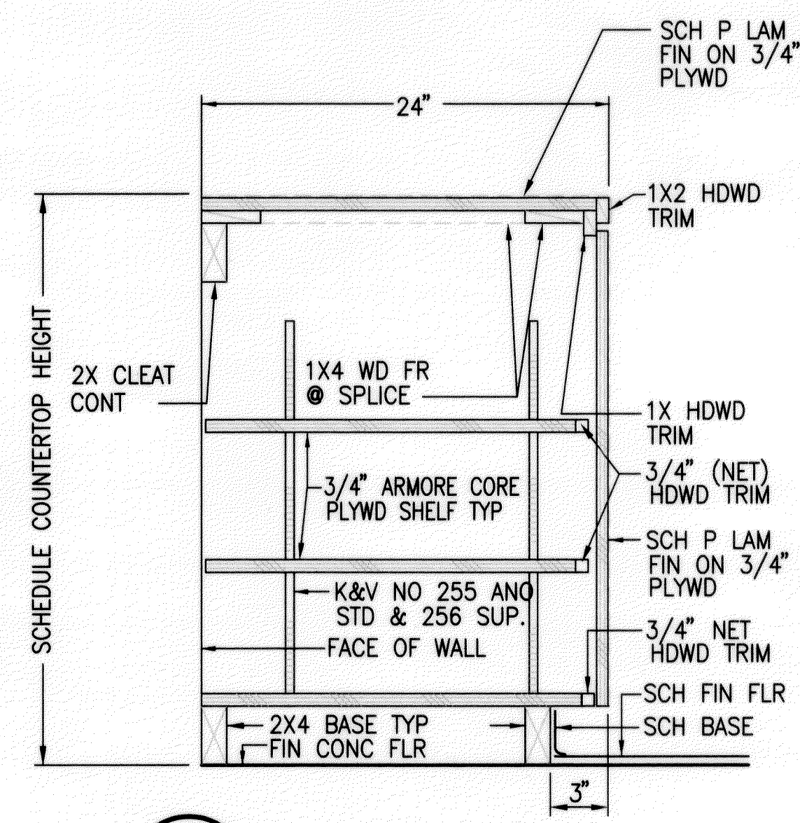
3 BASE CAB A7.4 SCALE: 1 1/2"=1'-0"
