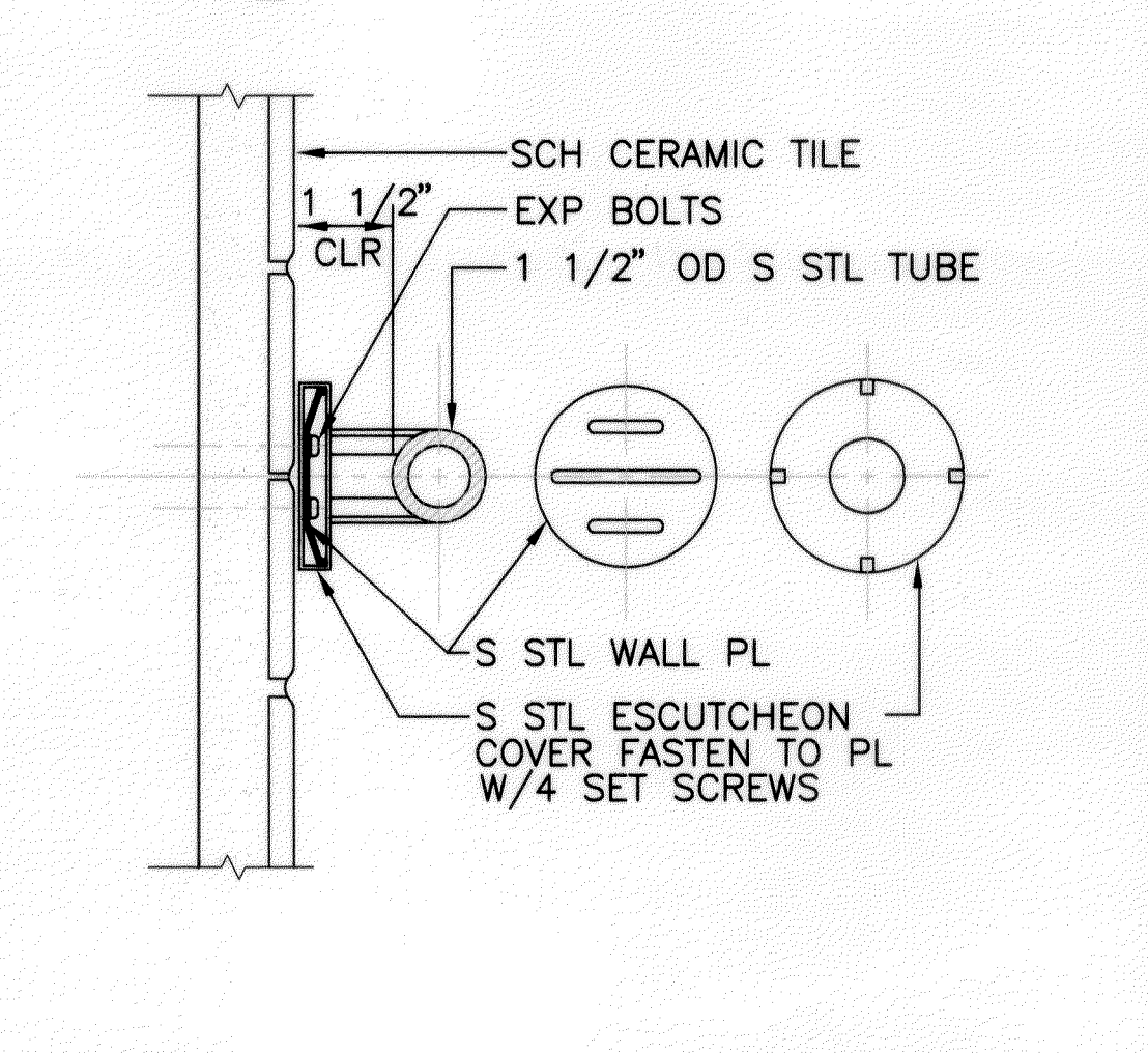
10 TOILET/GRAB BAR A7.4 SCALE: NTS
