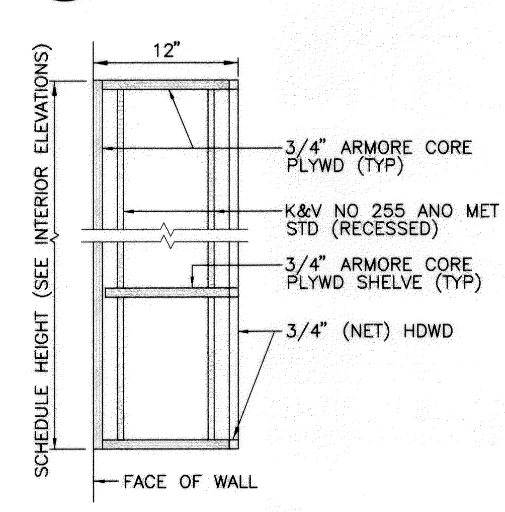
7 OPEN WALL CAB A7.4 SCALE: 1 1/2"=1'-0"
