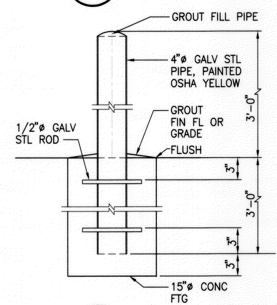
12 BOLLARD A7.4 SCALE: 1 1/2"=1'-0"
