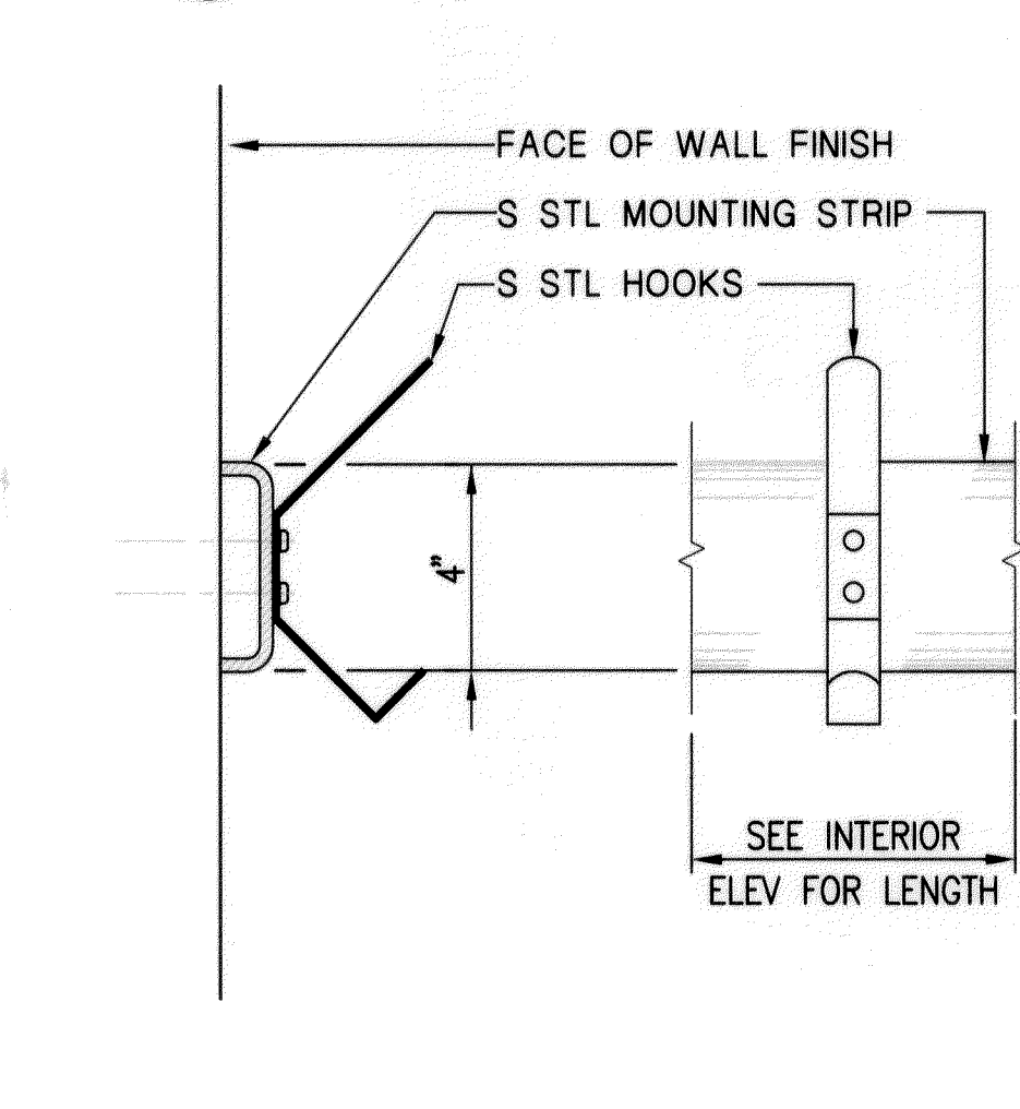
9 HOOK STRIP A7.4 SCALE: NTS
