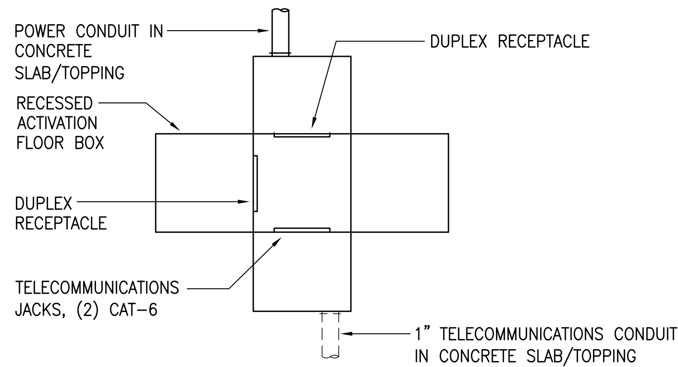
3 FLOOR OUTLET CONDUIT ROUTING E20 NO SCALE
