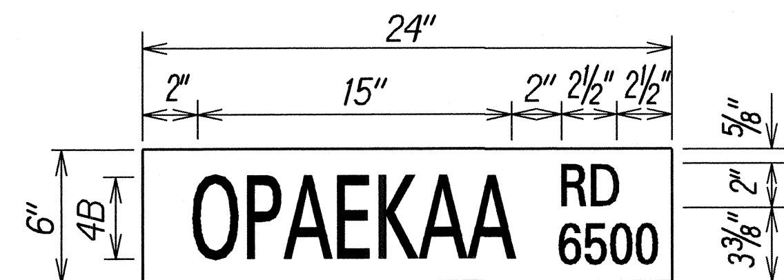
D3-1-5 Scale: 2" = 1'-0"
