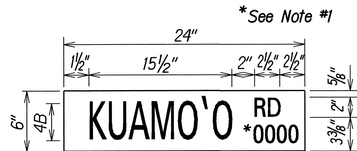
D3-1-1 Scale: 2" = 1'-0"
