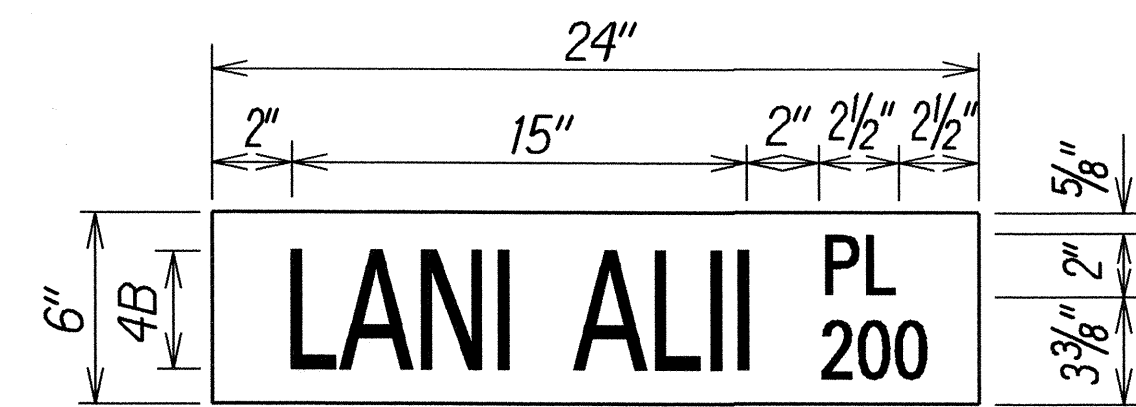
D3-1-12 Scale: 2" = 1'-0"
