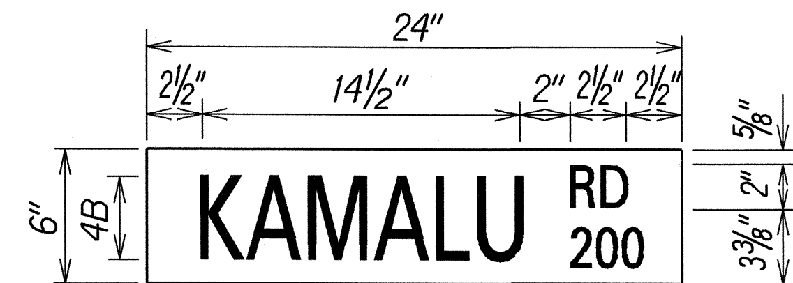
D3-1-10 Scale: 2" = 1'-0"
