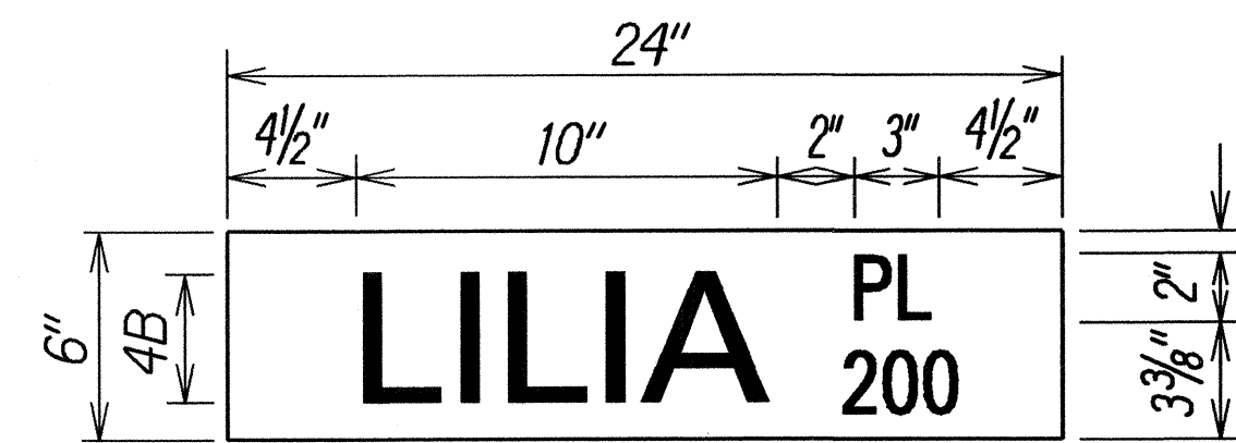
D3-1-18 Scale: 2" = 1'-0"
