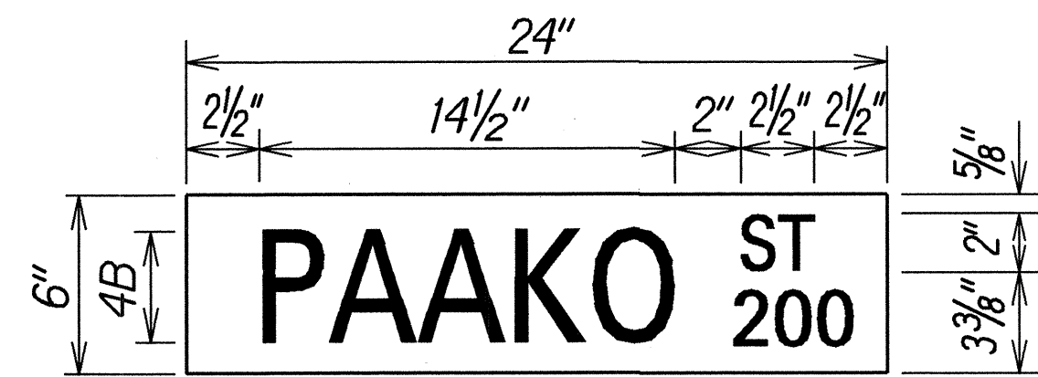
D3-1-2 Scale: 2" = 1'-0"
