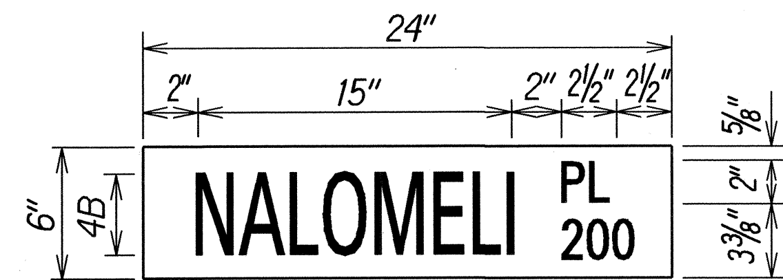
D3-1-6 Scale: 2" = 1'-0"
