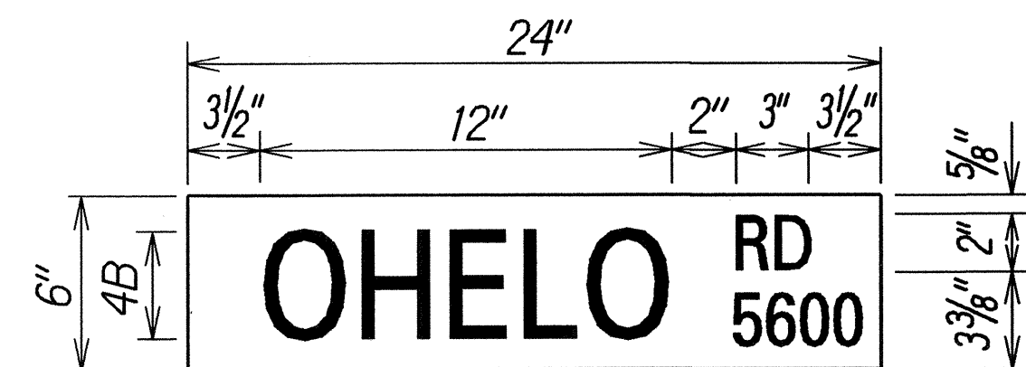
D3-1-17 Scale: 2" = 1'-0"
