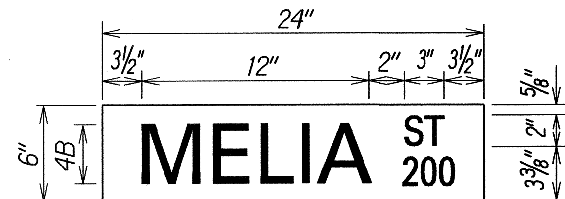
D3-1-15 Scale: 2" = 1'-0"
