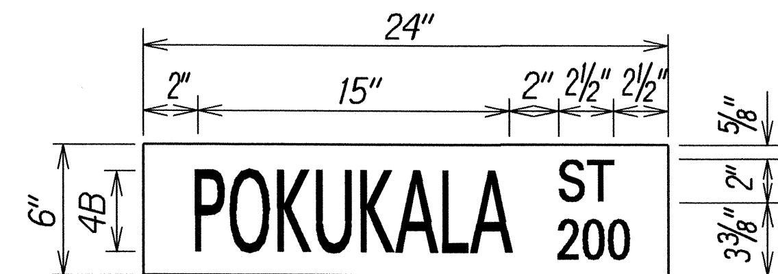
D3-1-9 Scale: 2" = 1'-0"
