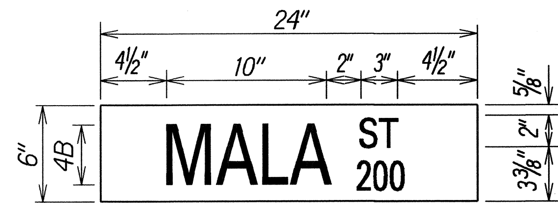
D3-1-14 Scale: 2" = 1'-0"
