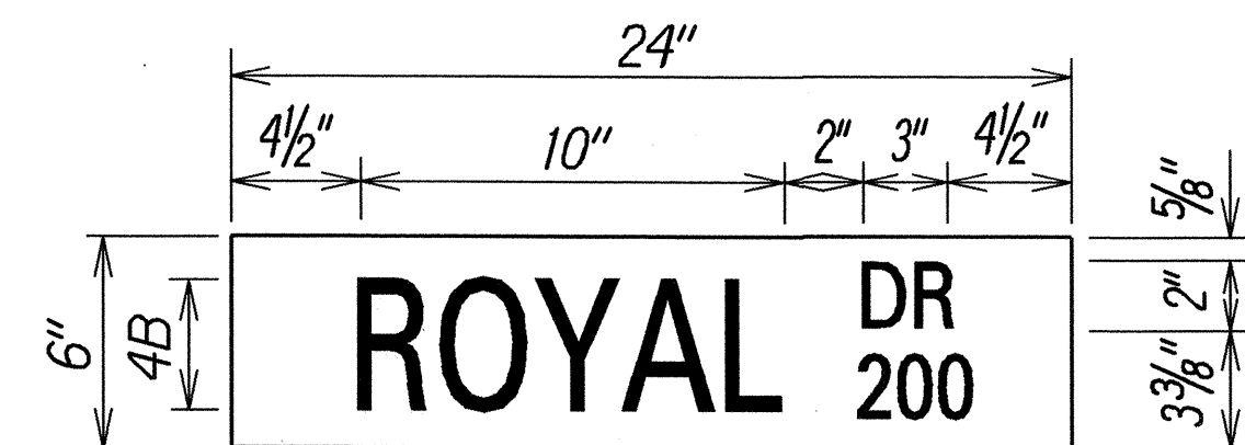
D3-1-11 Scale: 2" = 1'-0"
