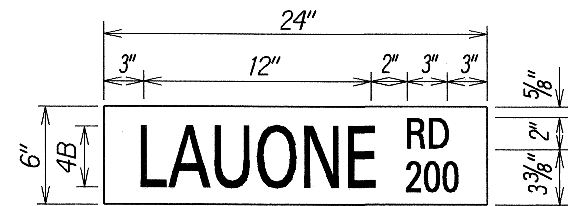
D3-1-8 Scale: 2" = 1'-0"
