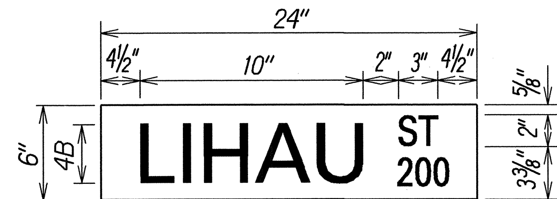
D3-1-4 Scale: 2" = 1'-0"
