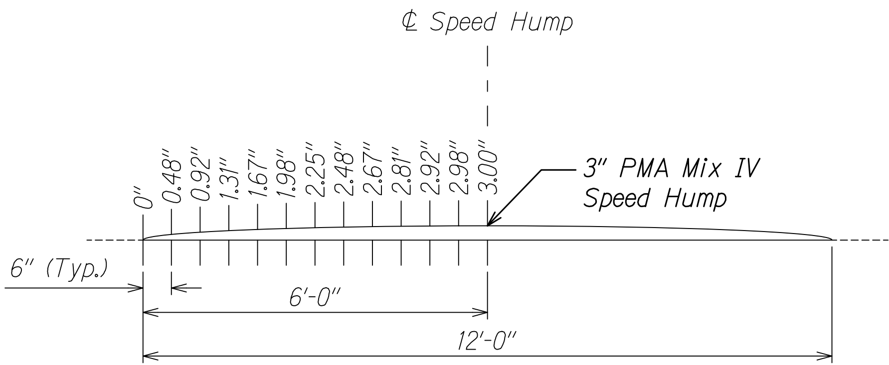
SECTION A-A C-21/C-21
