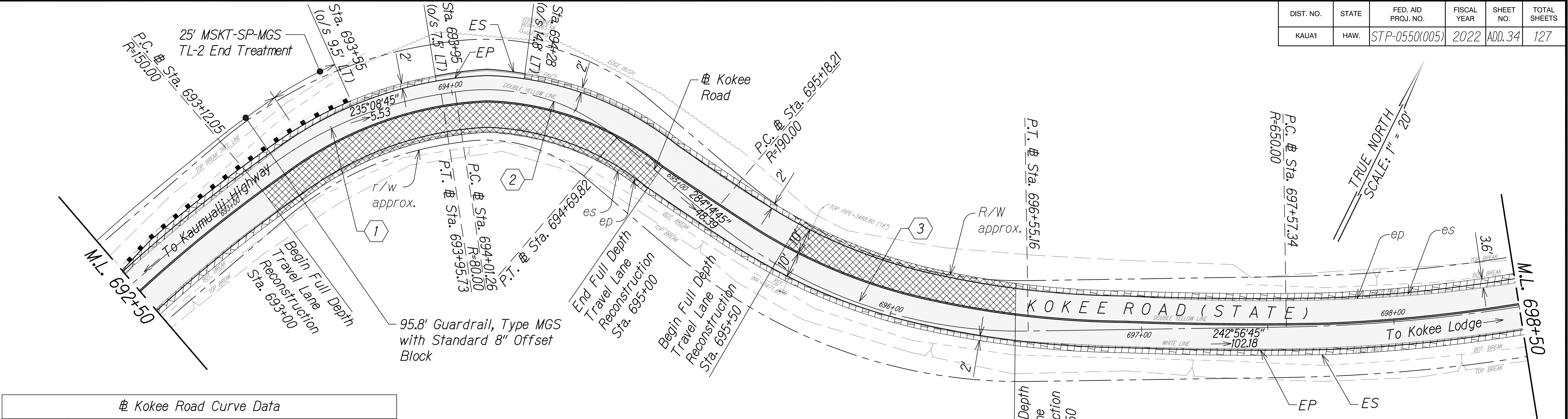
STA. 692+50 TO 698+50 (Kokee Road)
