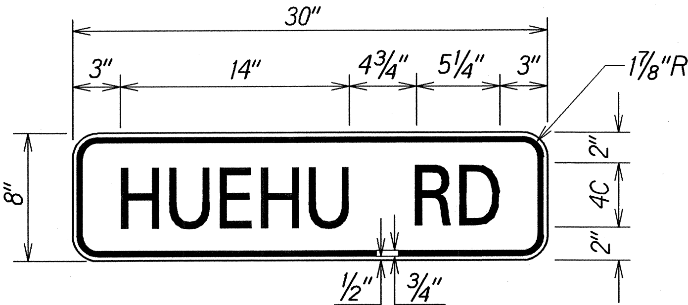
W16-8 Scale: 2" = 1'-0"
