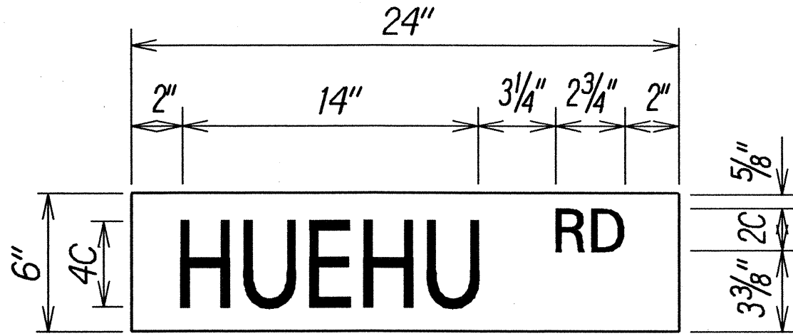
STREET NAME SIGN Scale: 2" = 1'-0"
