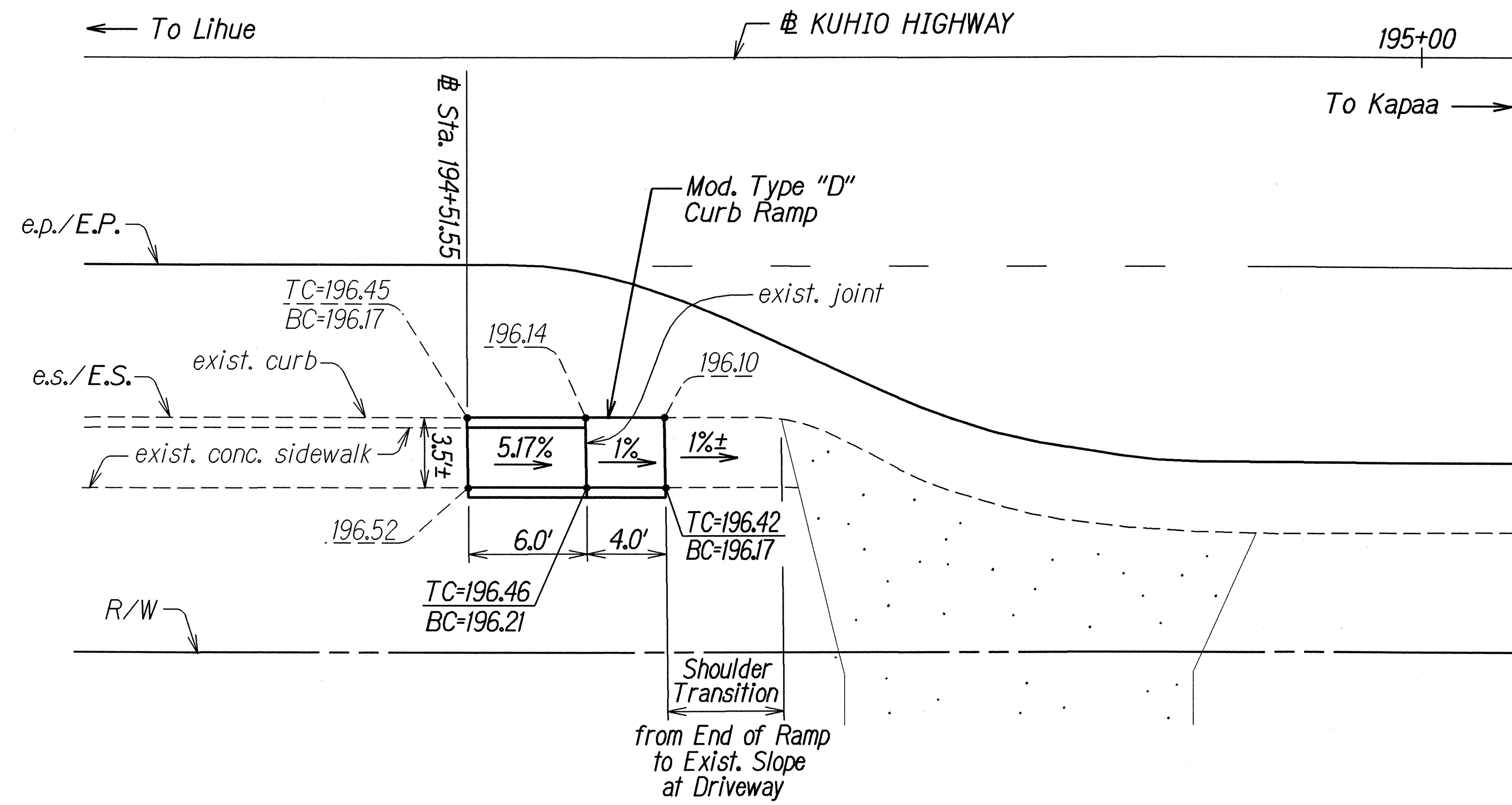
CURB RAMP #6 Scale: 1" = 5'
