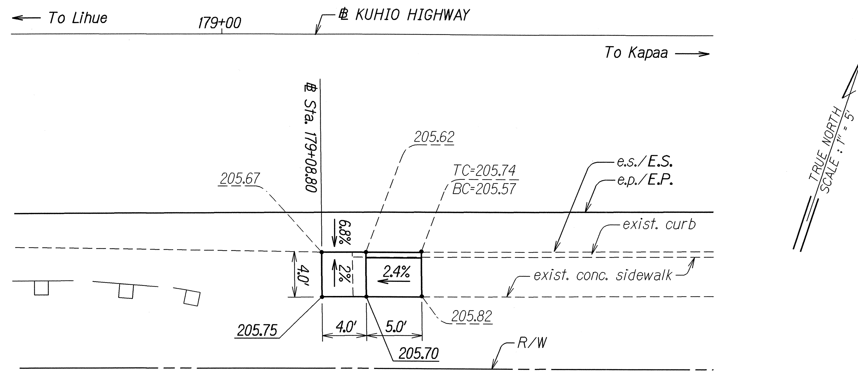
CURB RAMP #1 Scale: 1" = 5'
