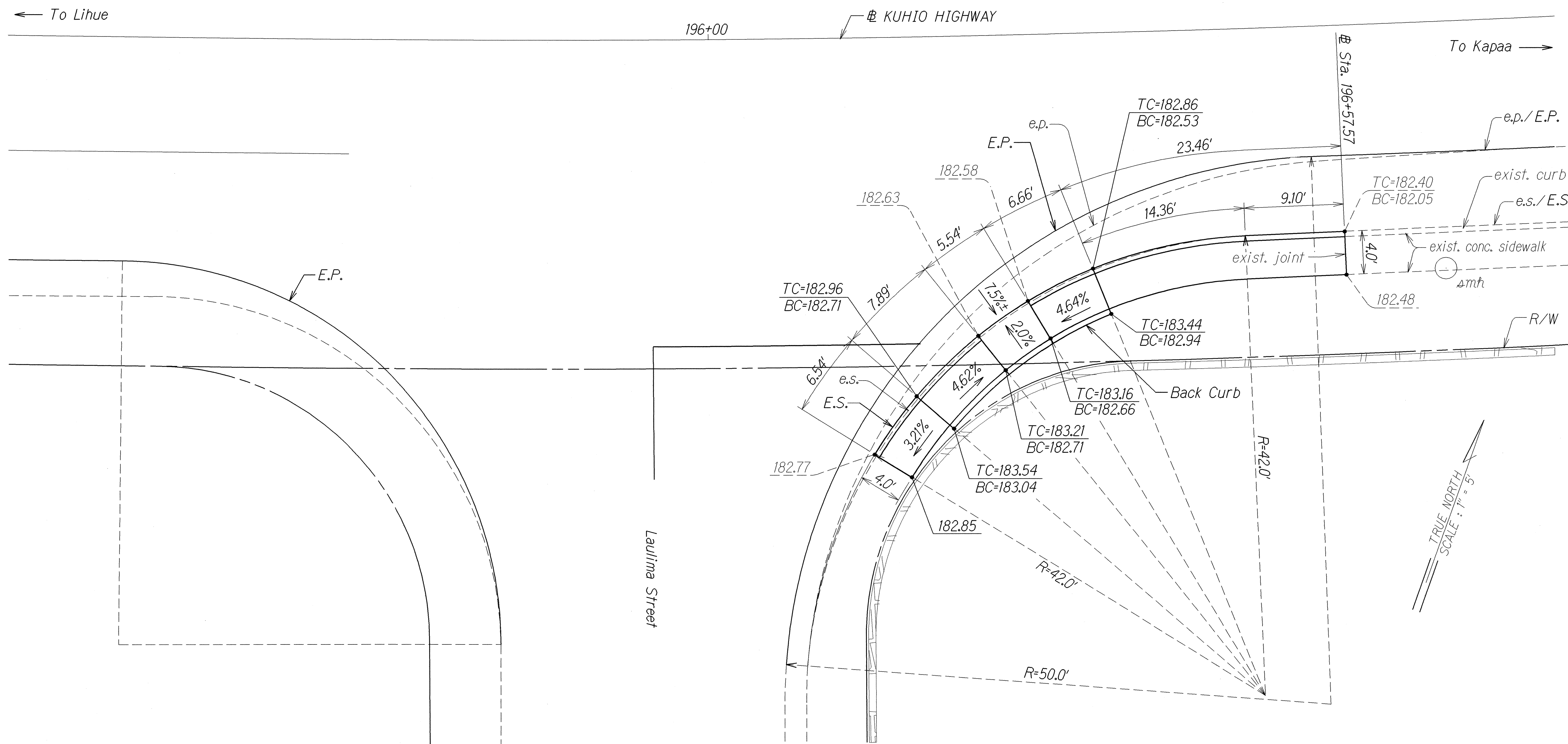
CURB RAMP #7 Scale: 1" = 5'
