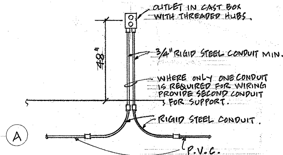
TYP. OUTLET DET. E3 N.T.S.
