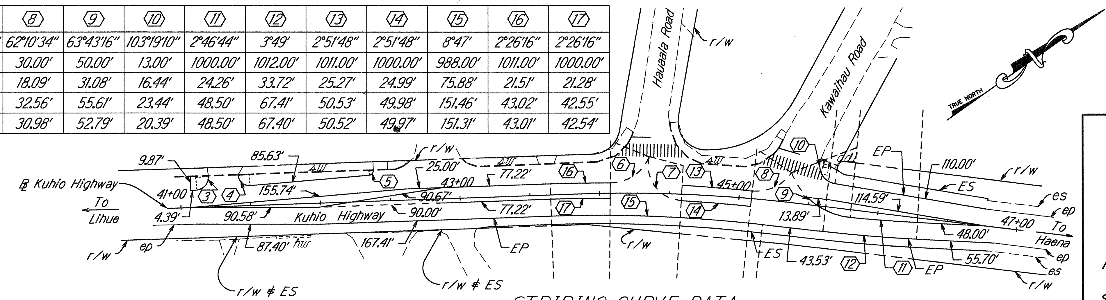
STRIPING CURVE DATA Scale: 1" = 40'
