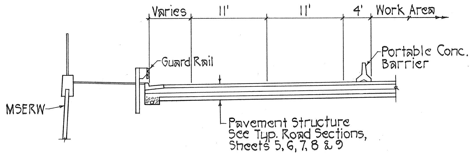
SECTION A Scale: 1"=8'
