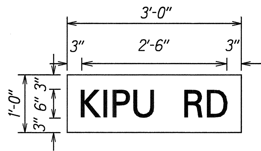
D1-1 Scale: 1"=1'
