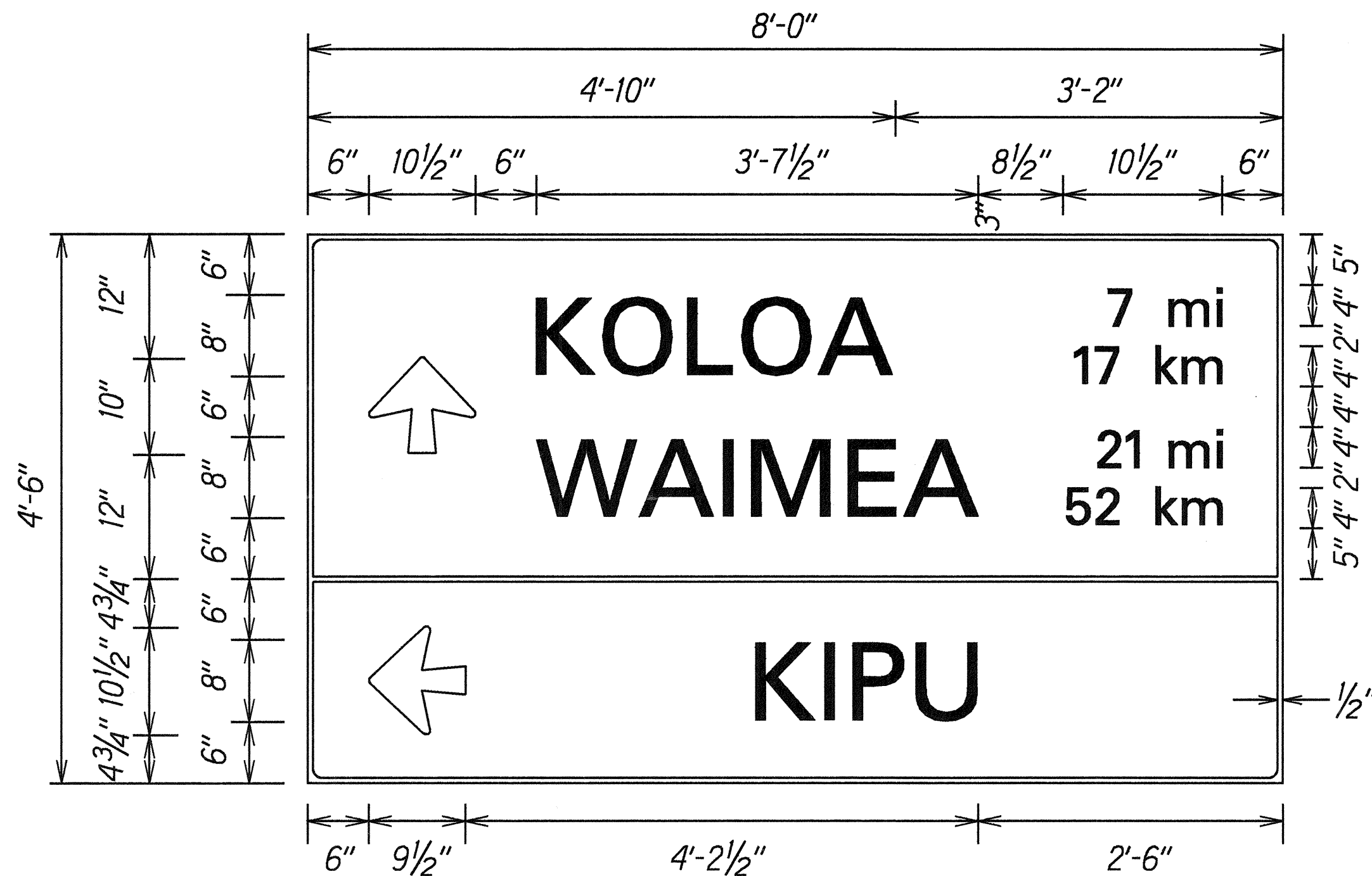
D1-2 Scale: 1"=1'
