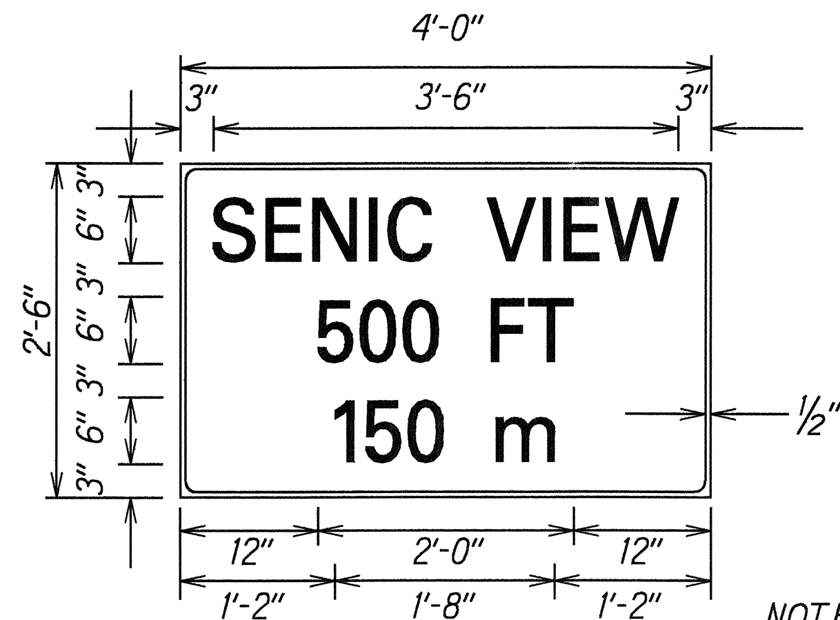
D6-2 Scale: 1"=1'
