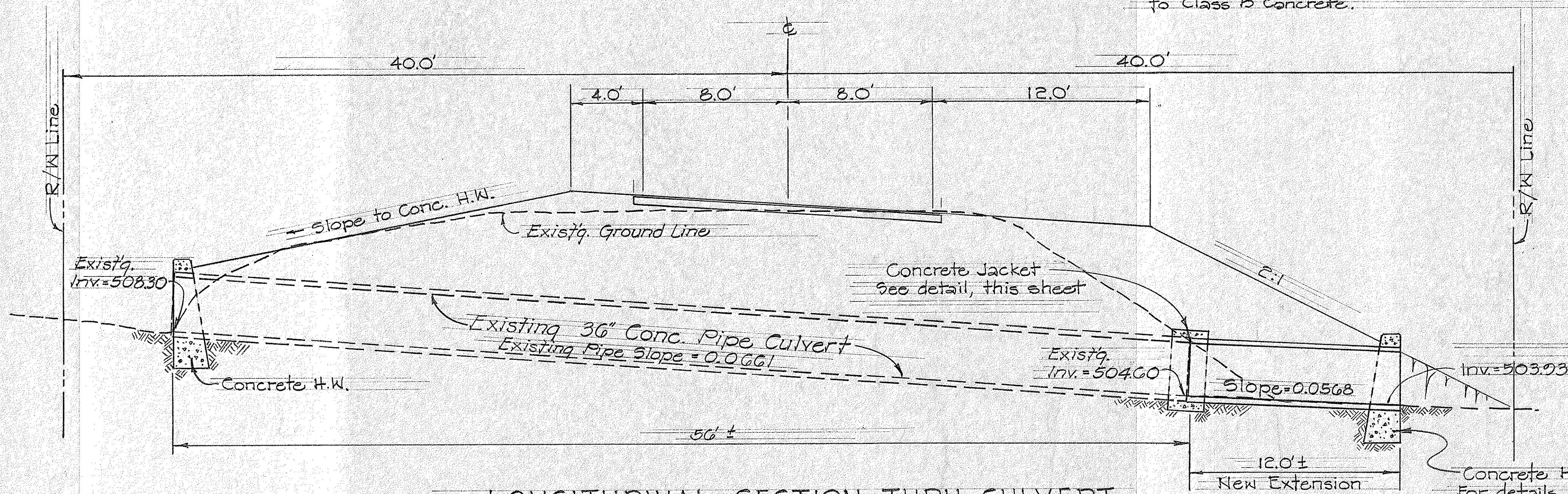
LONGITUDINAL SECTION THRU CULVERT AT STA. 145+71 Scale: 1/4" = 1'-0"
