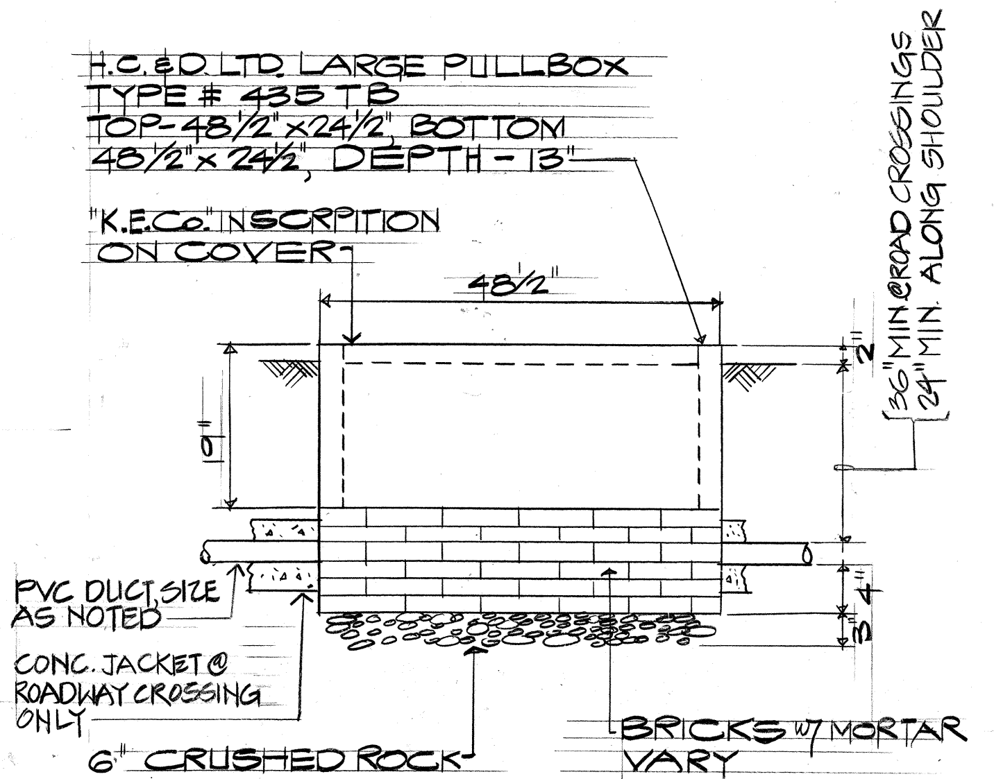
PULLBOX DETAIL E-3 N.T.S.
