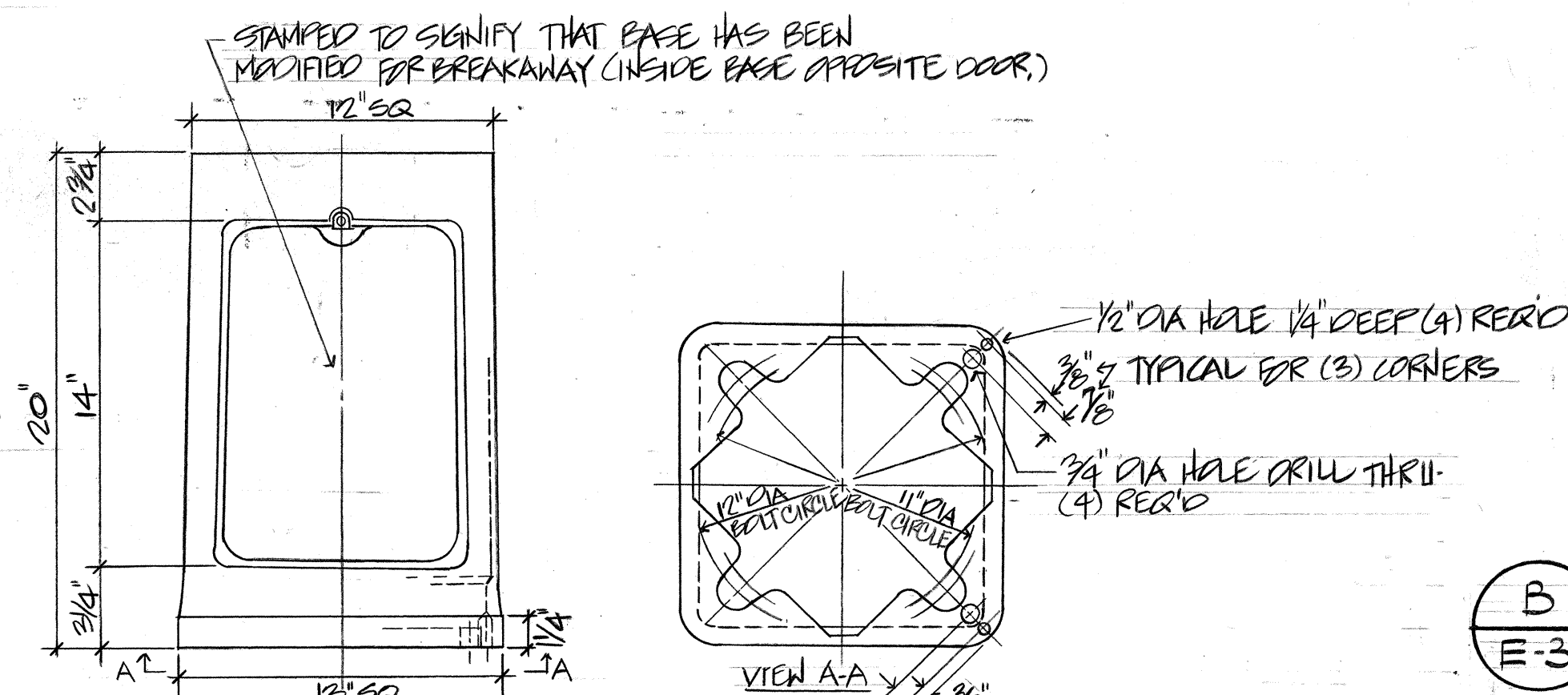
BREAKAWAY TRANSFORMER BASE E-3 N.T.S.
