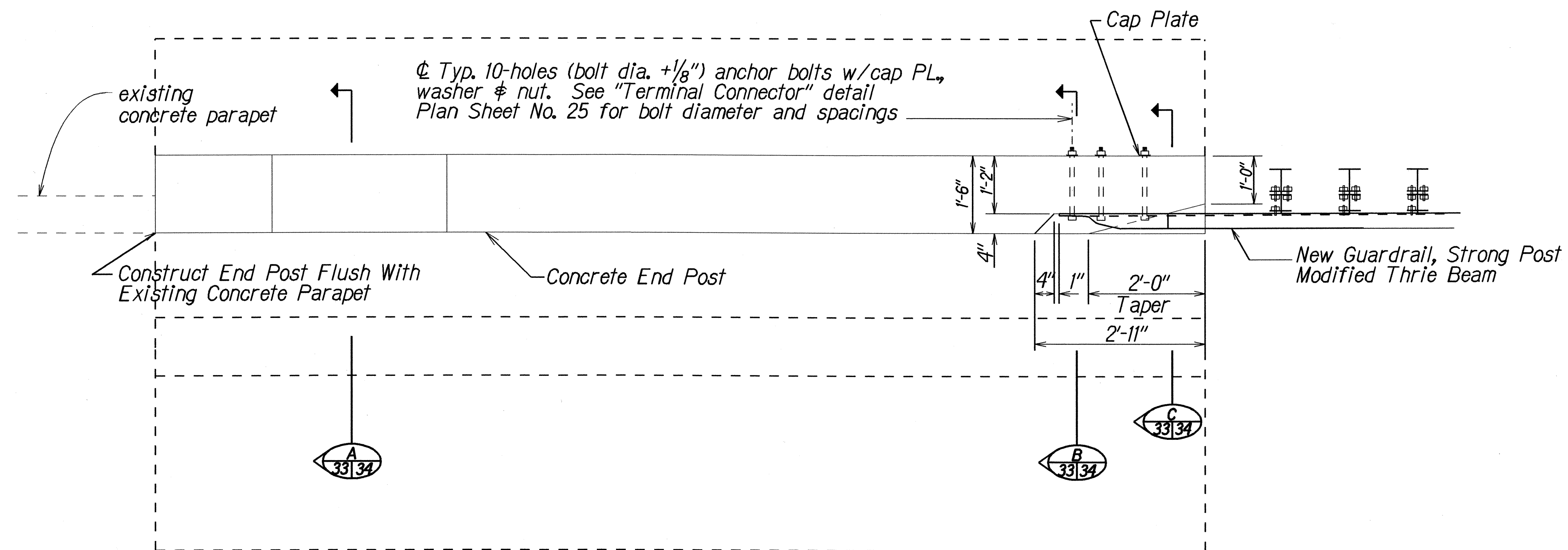
PLAN Scale: \frac{3}{4}" = 1'-0"
