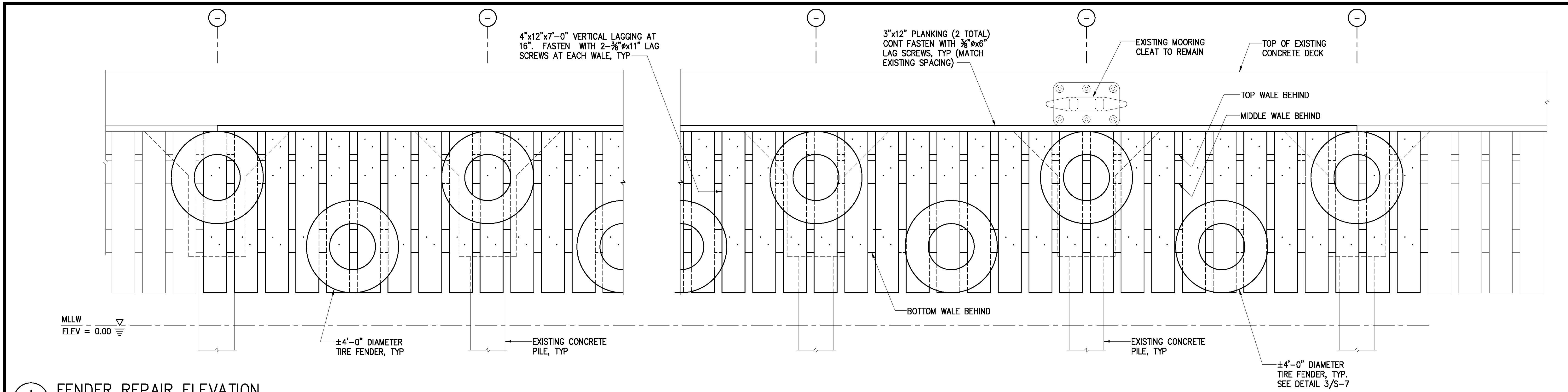
1 FENDER REPAIR ELEVATION S-6 SCALE: 1/2" = 1'-0"
