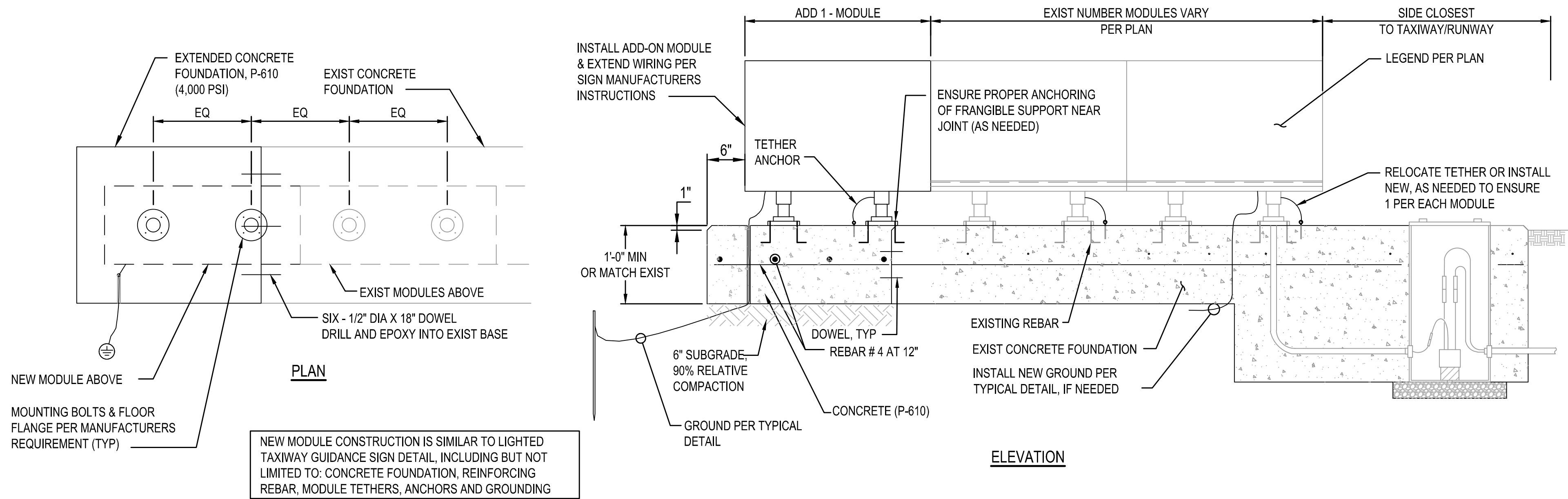
EXISTING SIGN PAD MODIFICATION DETAIL SCALE: N.T.S.
