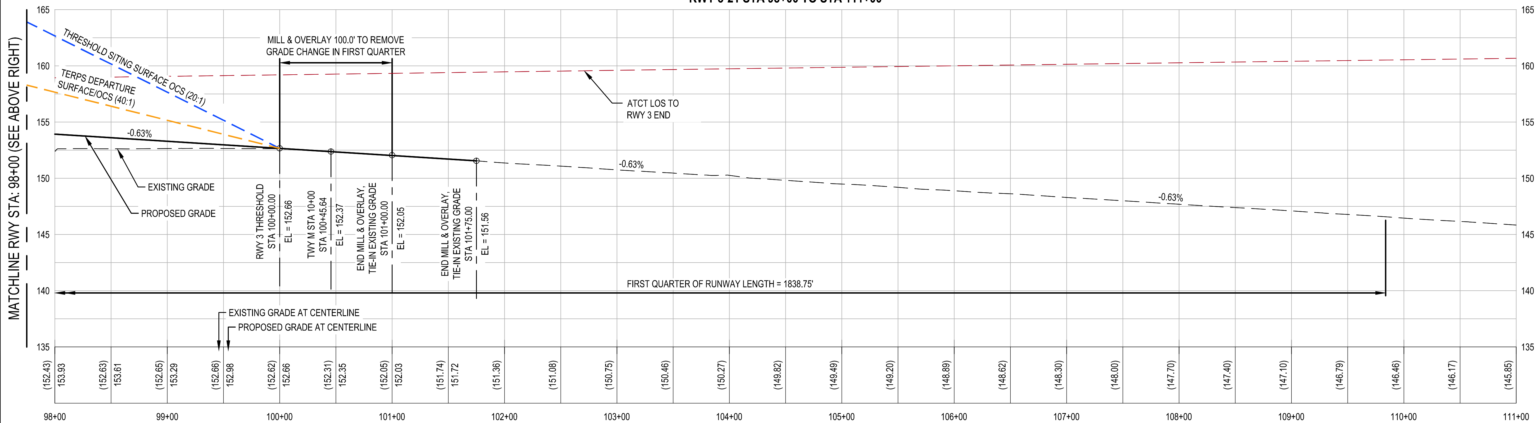
RUNWAY 3 - PROFILE STA 98+00 TO STA 111+00
