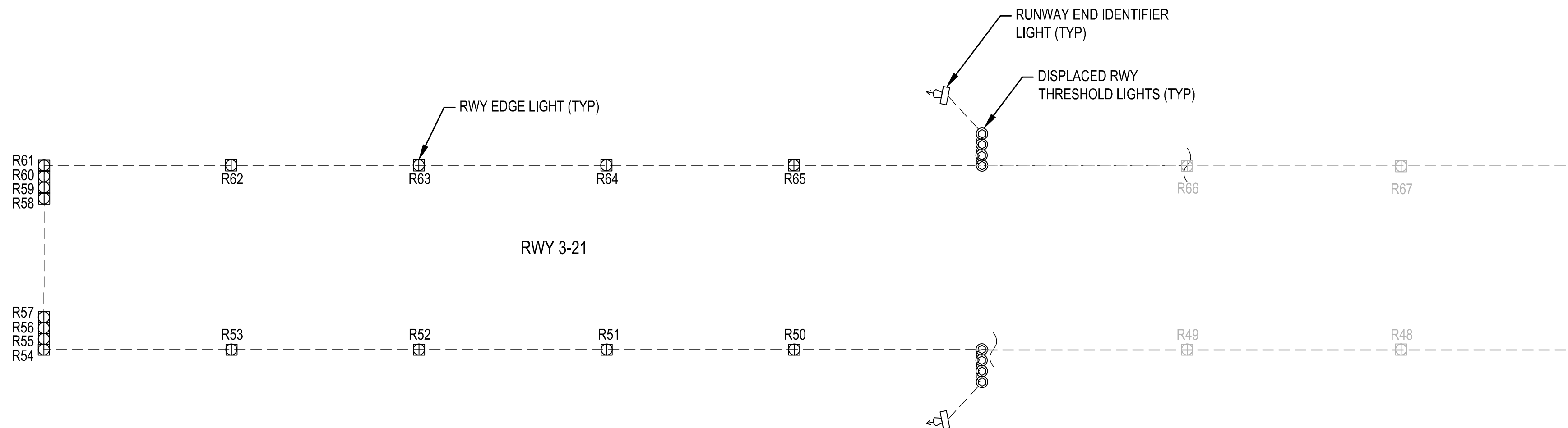
PARTIAL CIRCUIT DIAGRAM - RUNWAY R-2 SCALE: N.T.S.
