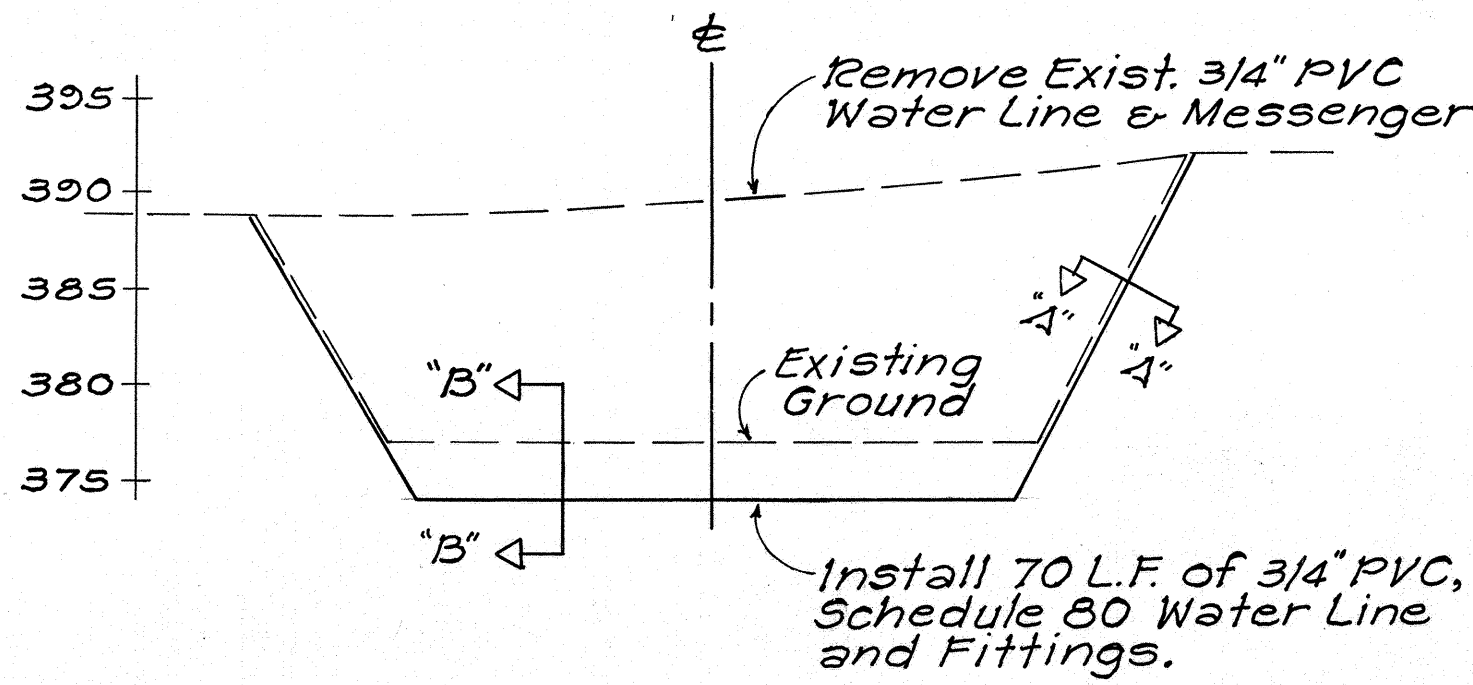
WATER LINE @ STA. 101+34 ± (N.T.S.)
